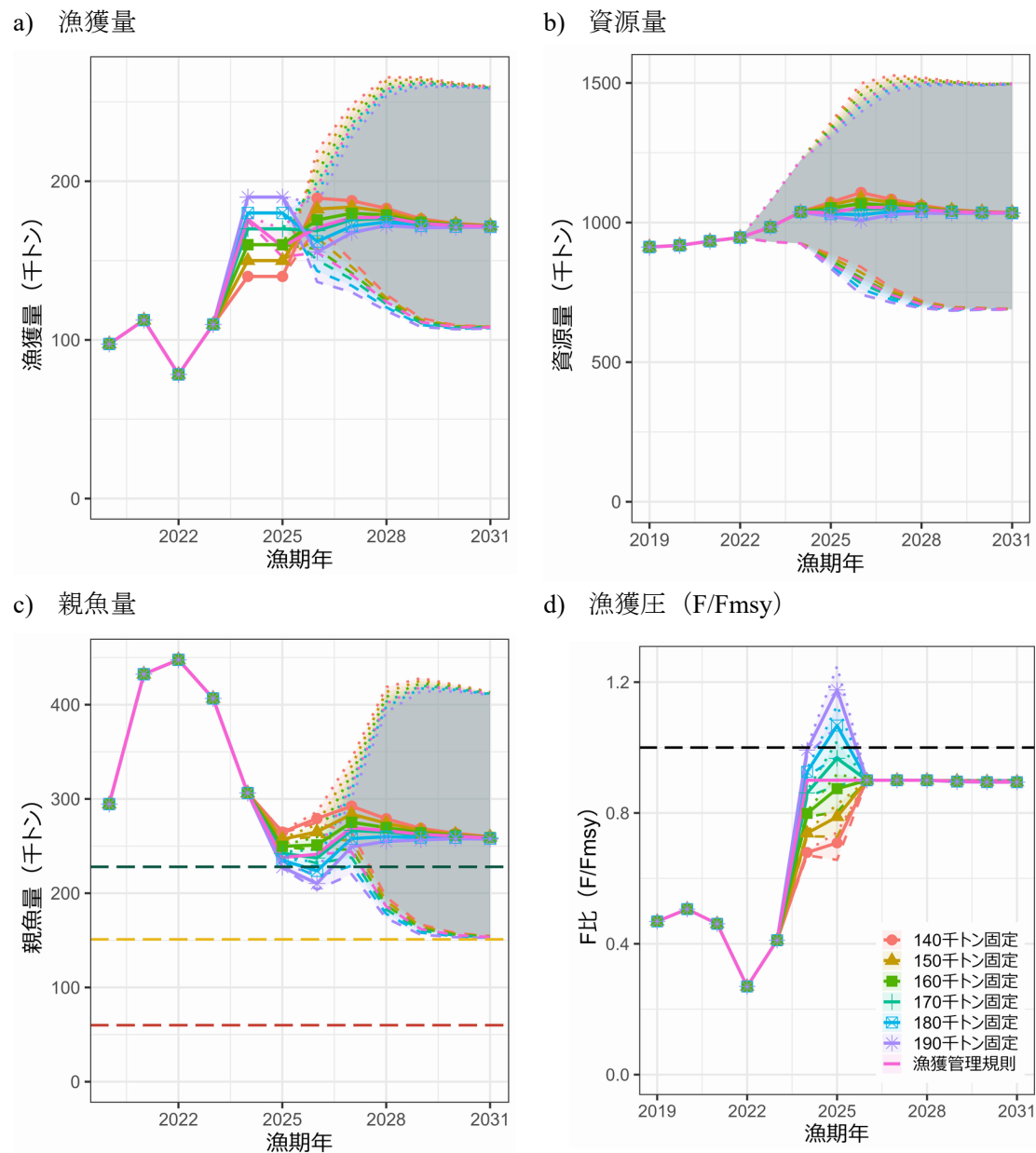
図 1. 漁獲量を 140 千～190 千トンで 2 年間固定した場合と漁獲管理規則 ( \beta=0.9 ) で漁獲を続けた場合とでの将来予測の比較
