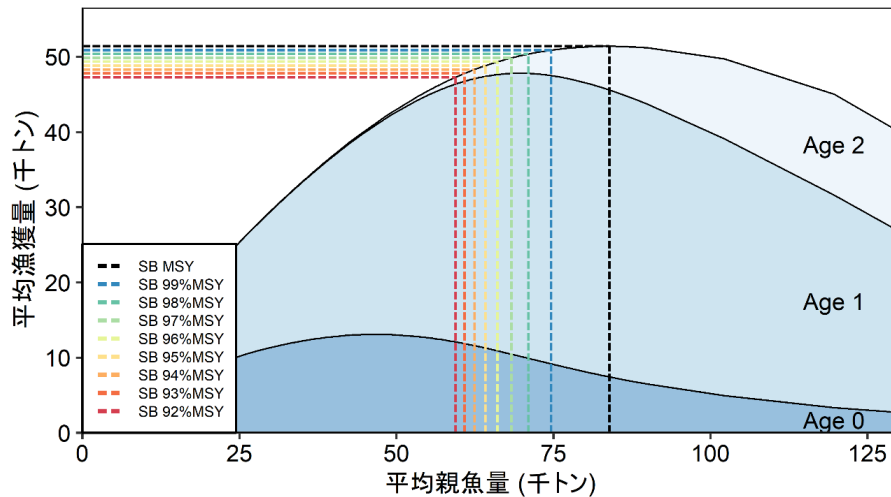
図 1. 平衡状態における平均親魚量と年齢別平均漁獲量および SB_{99\%msy} ～ SB_{92\%msy} との関係（漁獲量曲線）
