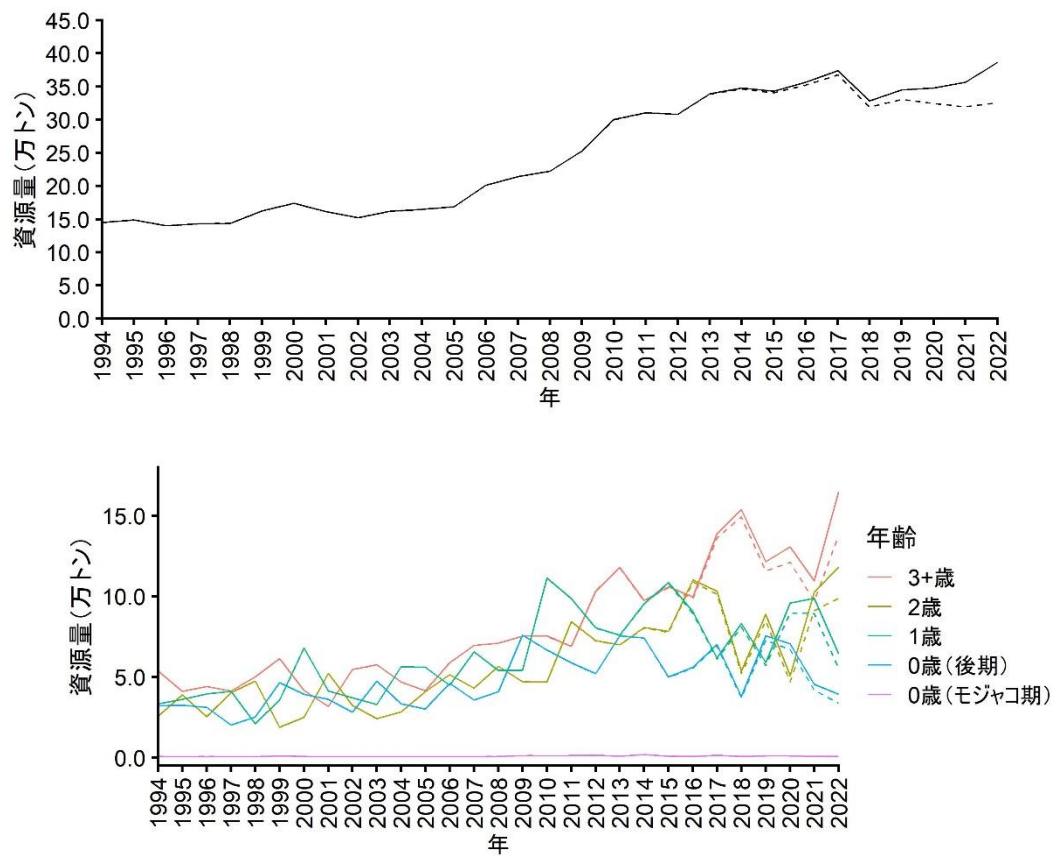
図3. チューニング VPA による資源評価結果への影響 (資源量)
