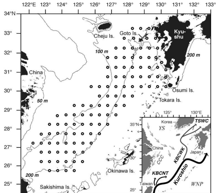
図1. ニューストンネットを用いた新規加入量調査の測点 (Sassa et al. 2020 改変) 丸は各観測点、破線は水深を示す。
