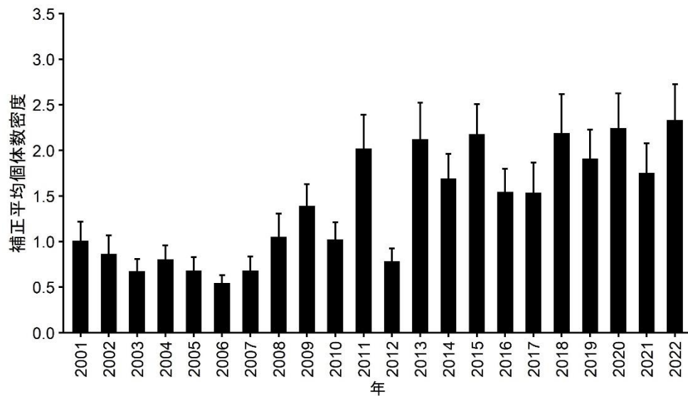
図2. ブリ仔魚の補正平均個体密度の推移 エラーバーは標準誤差を示す。
