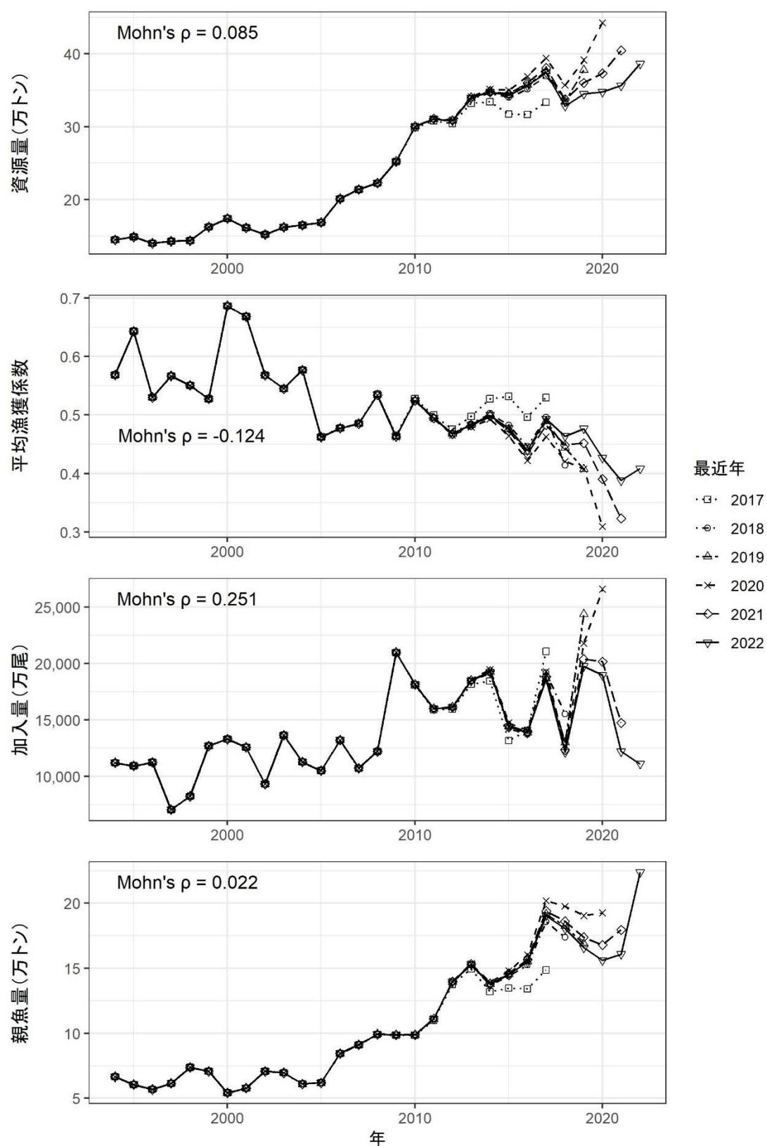
図6. レトロスペクティブ解析 (チューニング VPA) Mohn's \rho の値は資源尾数では各年齢の平均を示す。
