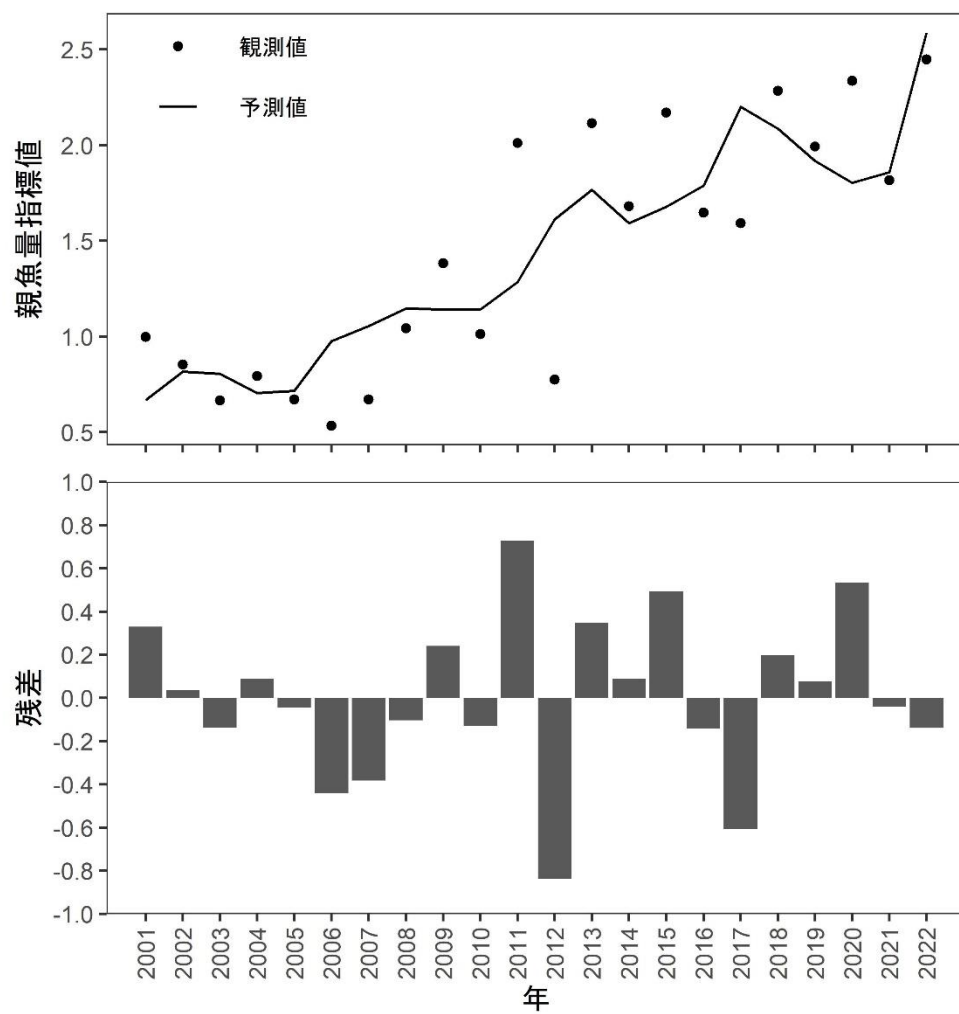
図 5. チューニング VPA による親魚量指標の予測値と観測値の推移（上段）と残差（下段）の推移 図中の折れ線は予測値、黒丸は観測値を示す。
