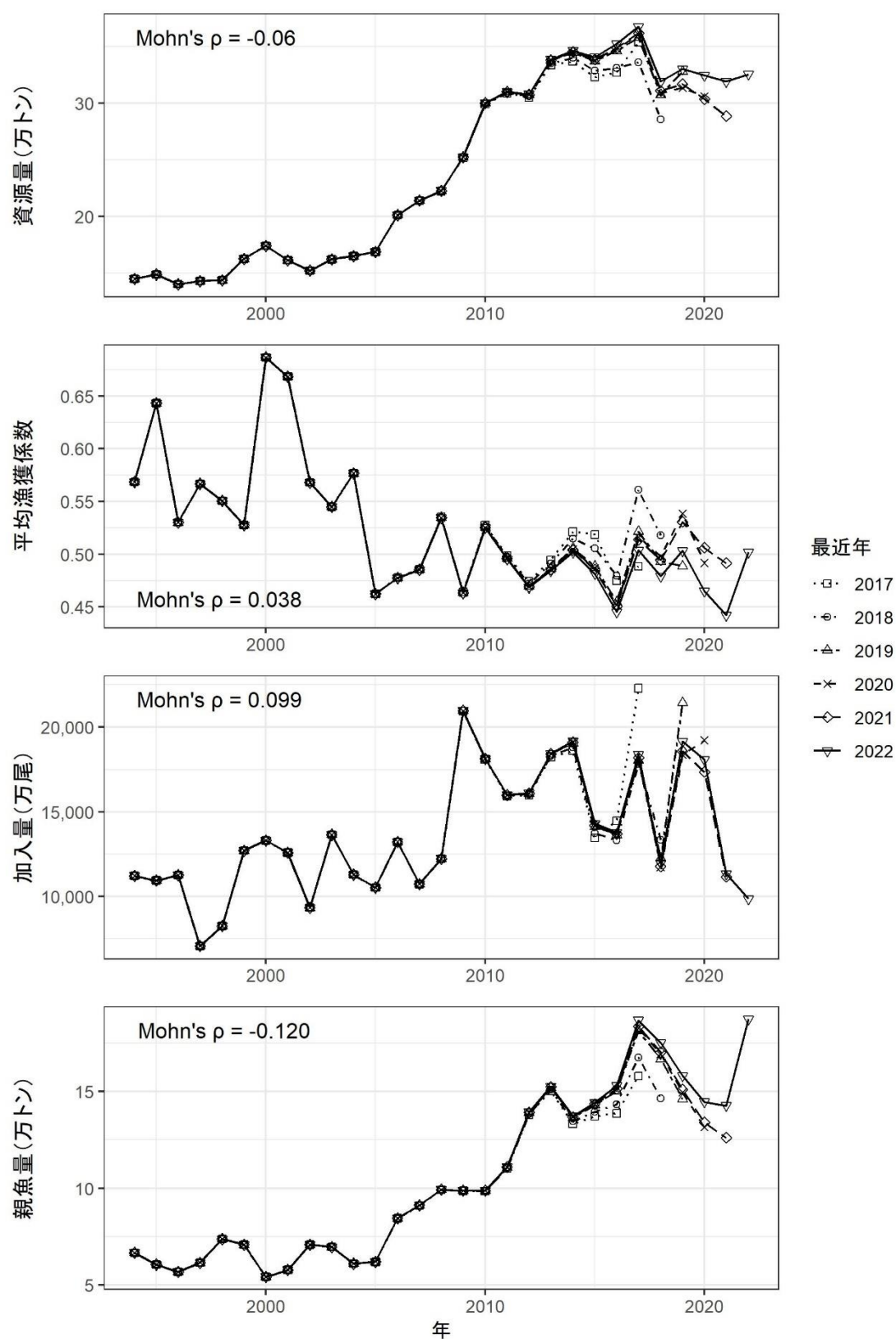
図7. レトロスペクティブ解析 (従来 VPA)
