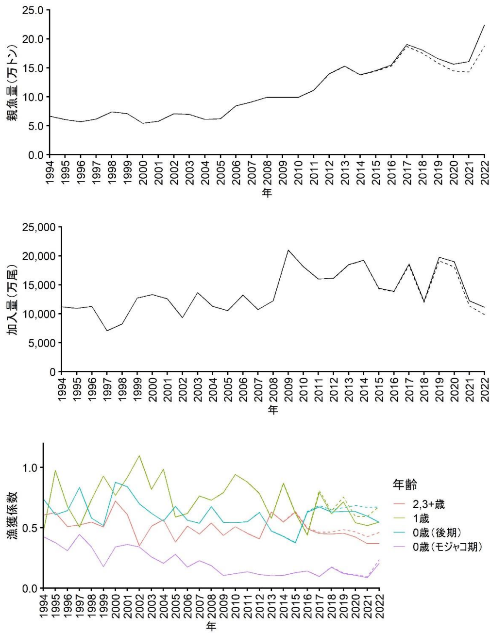
図 4. チューニング VPA による資源評価結果への影響（加入量、親魚量、漁獲係数）
