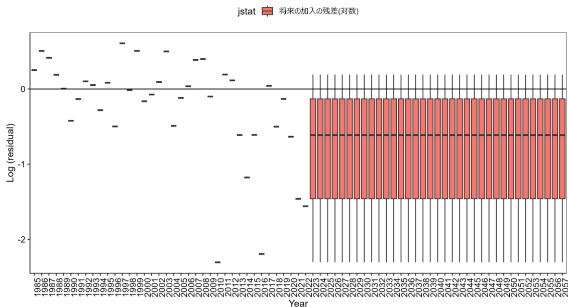
補足図 2-1. ホッケー・スティック型再生産関係式を最小絶対値法で当てはめた場合の加入量の予測値に対する観測値の残差（1985～2022 年）と将来予測において用いた残差（2010～2022 年の残差リサンプリング）
