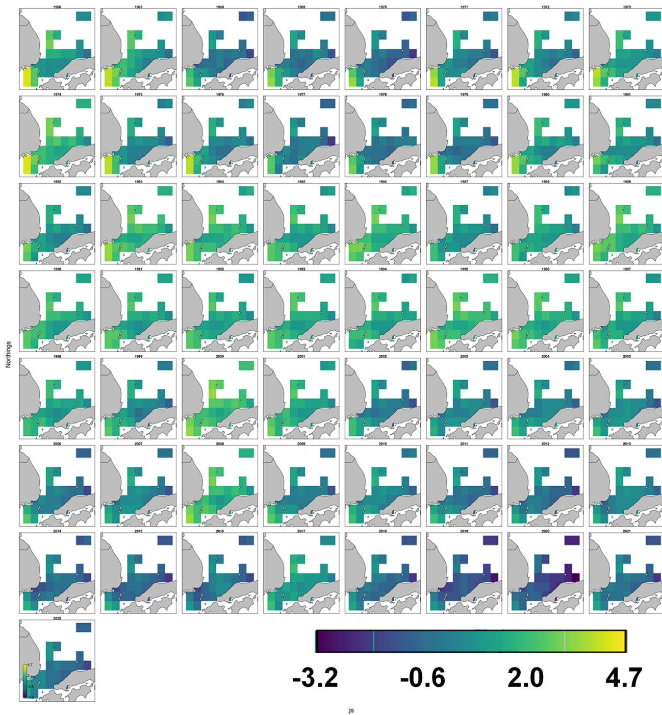
図3. 各年の資源量指数の空間分布 色は資源量指標値の多寡を示す。
