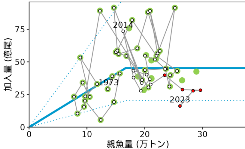
図7 再生産関係
