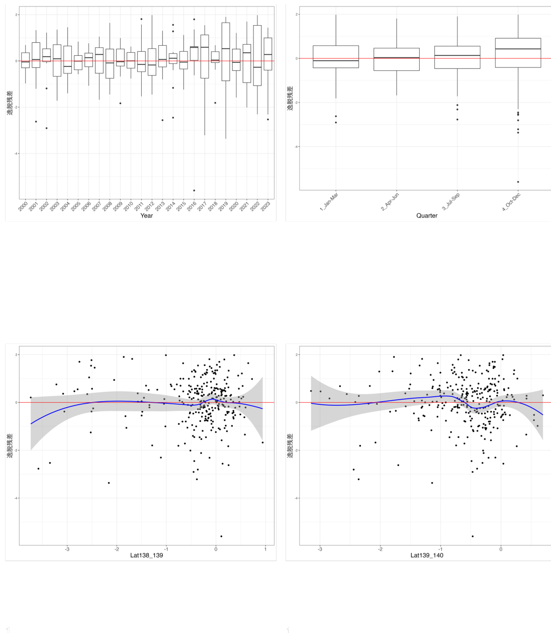
図 6. ベストモデルの層別逸脱残差 Lat138_139、Lat139_140 に関する残差図の青線と灰帯は、残差にフィッティングさせた平滑化曲線 (loess) と、その 95%信頼区間を示す。
