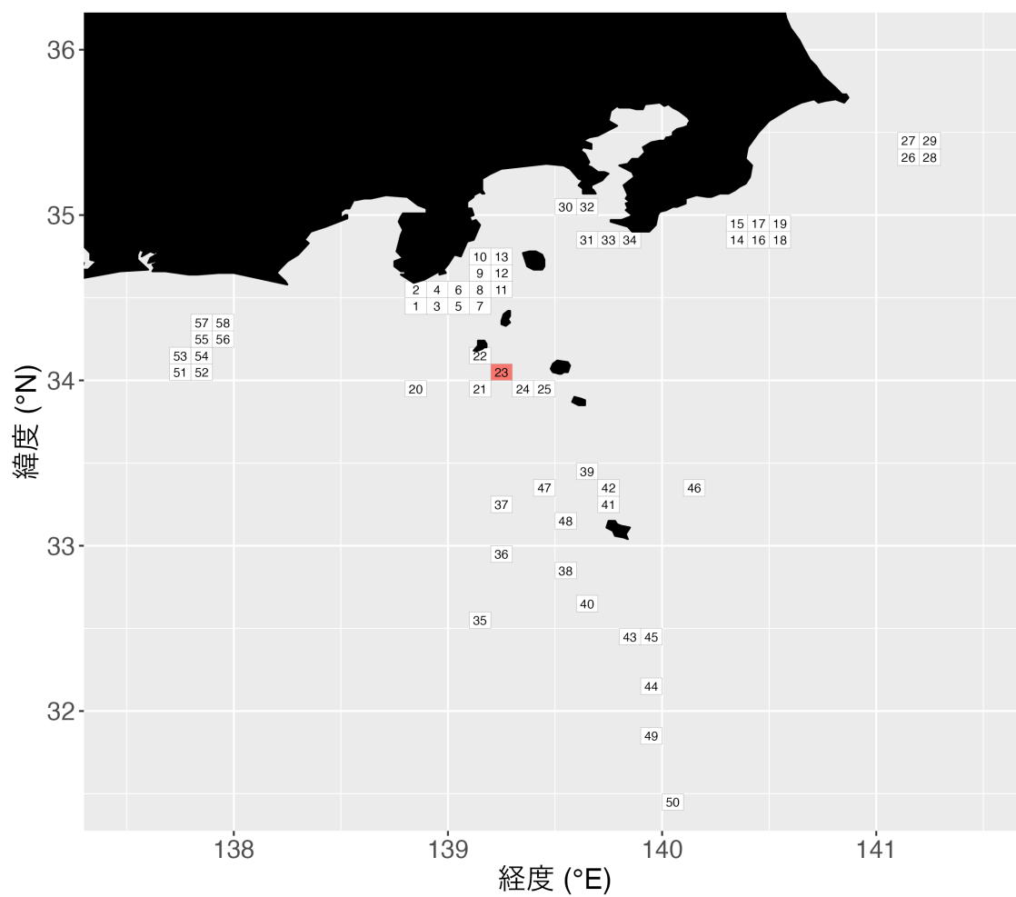
図 1. FRA-ROMS II再解析値の抽出に用いた各地区の漁場範囲 緯度経度 0.1°グリッドごとにデータを抽出。神津島地区は23番のグリッドを使用。
