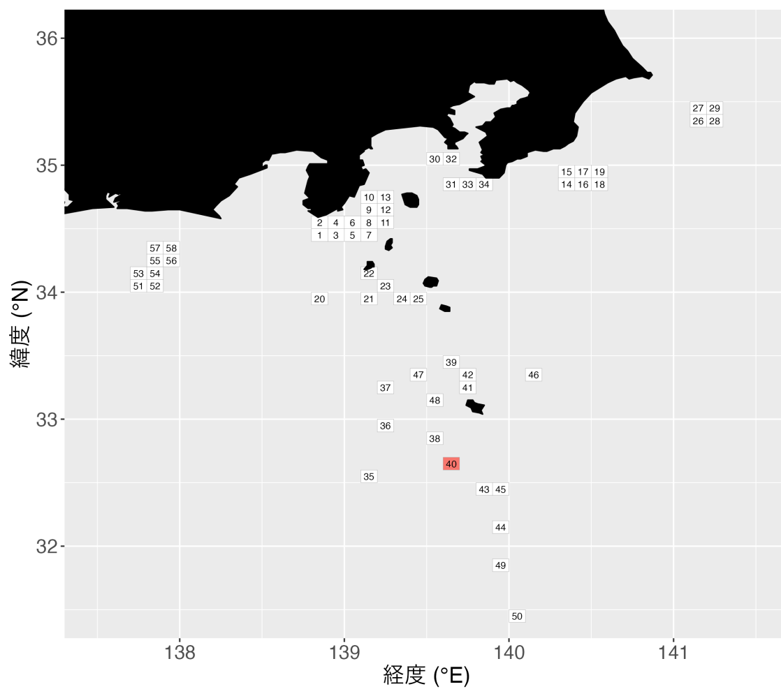
図 1. FRA-ROMS II再解析値の抽出に用いた各地区の漁場範囲 緯度経度 0.1°グリッドごとにデータを抽出。八丈島地区は 40 番のグリッドを使用。
