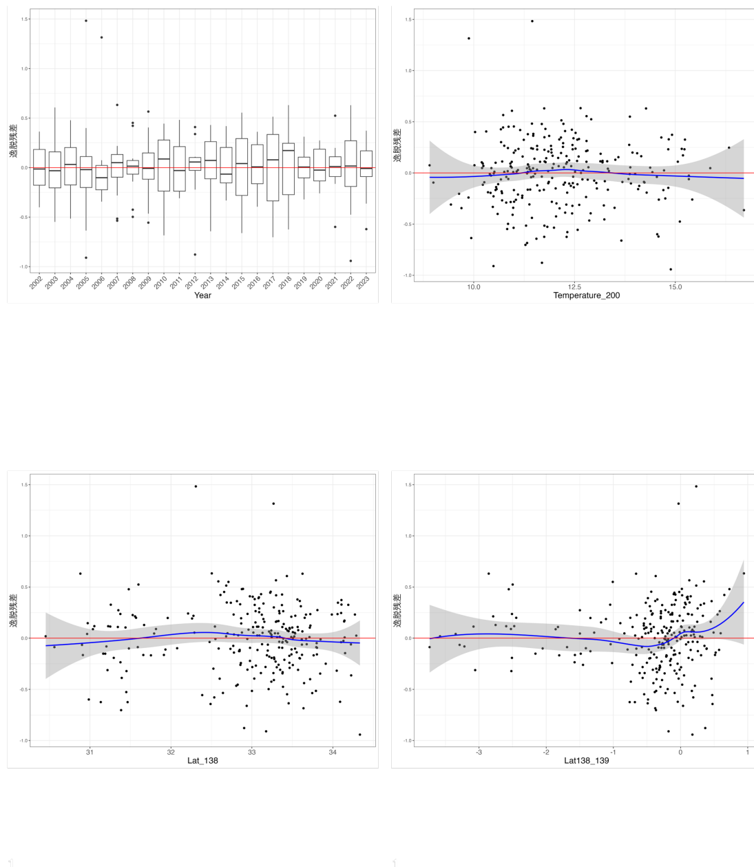
図 6. ベストモデルの層別逸脱残差 Temperature_200、Lat_138、Lat138_139 に関する残差図の青線と灰帯は、残差にフィッティングさせた平滑化曲線 (loess) と、その 95%信頼区間を示す。
