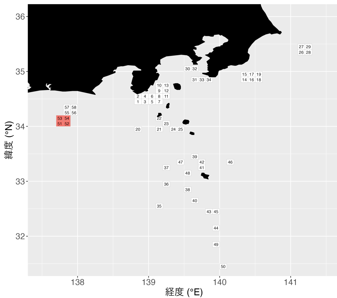
図 1. FRA-ROMS II再解析値の抽出に用いた各地区の漁場範囲 緯度経度 0.1°グリッドごとにデータを抽出。御前崎地区は 51～54 番のグリッドを使用。
