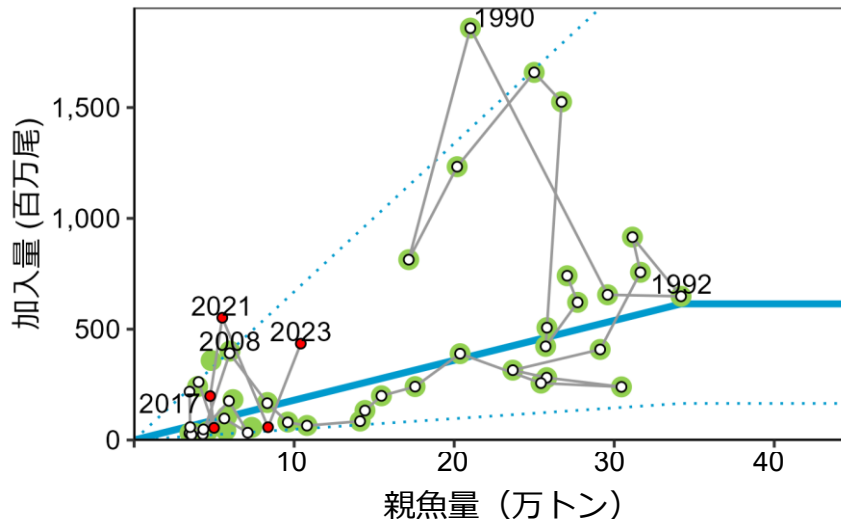
図6 再生産関係
