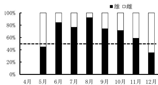
図 5-2 性比(佐賀県)
