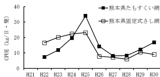
図2－2 CPUEの推移
