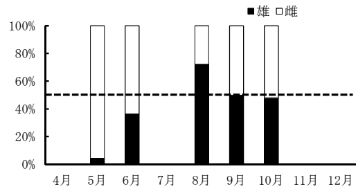
図 5-4 性比(熊本県)
