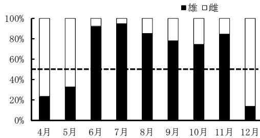
図 5-1 性比(福岡県)
