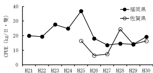
図2－1 CPUEの推移
