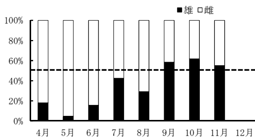
図 5-3 性比(長崎県)
