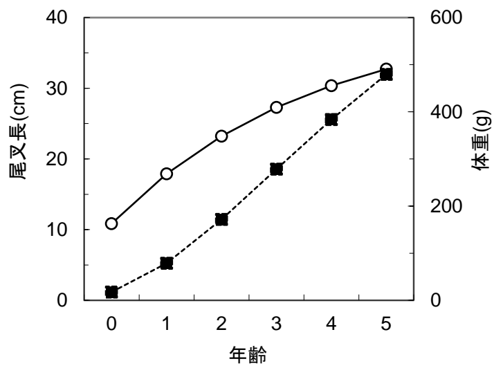
図 2-2. 年齢と成長
