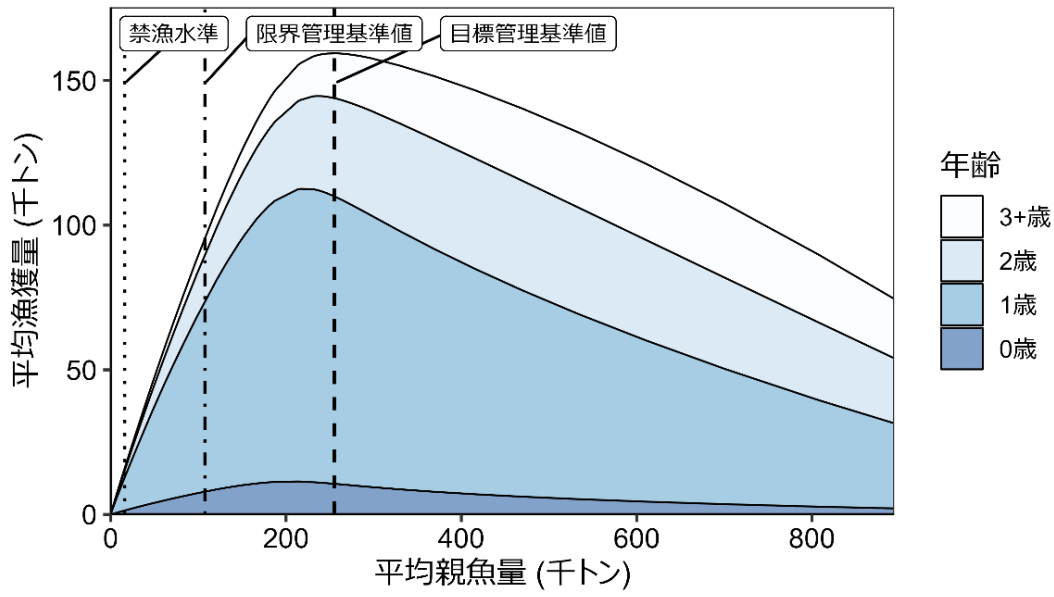
図 4-15. 漁獲量曲線
