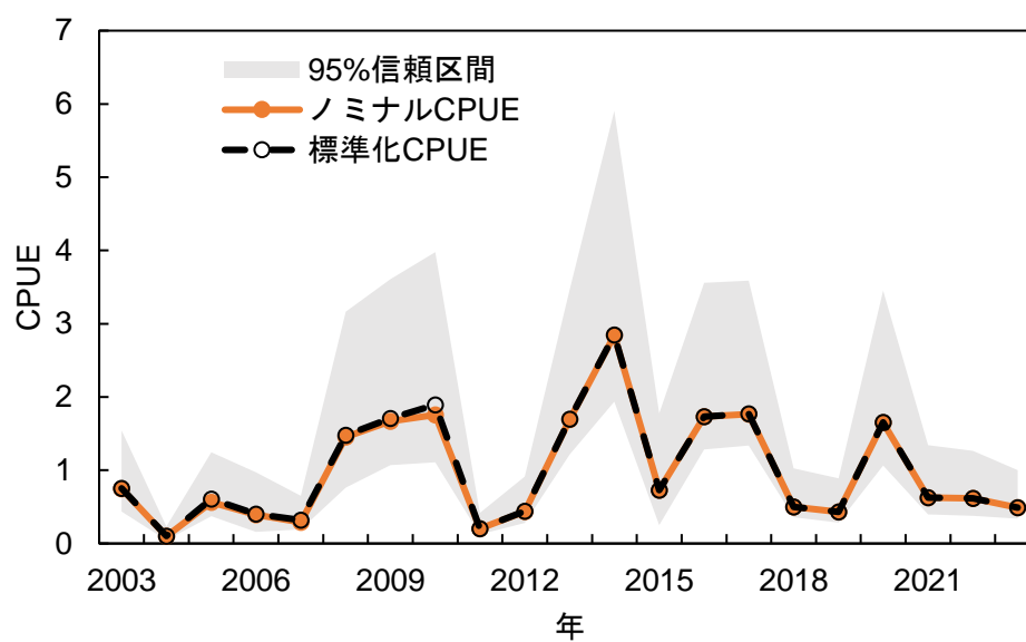
補足図 5-2. 新規加入量調査のノミナル CPUE と標準化 CPUE および 95%信頼区間の推移 それぞれの平均値で割り、規格化した。
