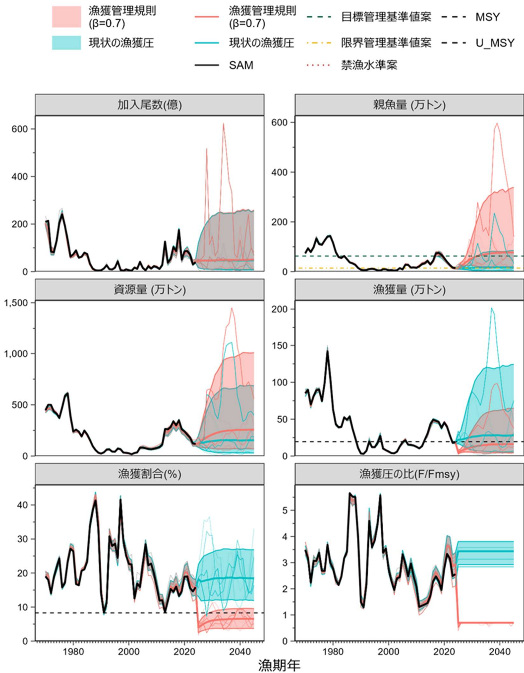
補足図 4-2. 漁獲管理規則案に従って漁獲を続けた場合（赤線）と現状の漁獲圧（F2021-2023）で漁獲を続けた場合（青線）の将来予測 太実線は中央値、網掛けはシミュレーション結果の 90%が含まれる予測区間、細線は 5 通りの将来予測の例示である。親魚量の図の緑破線は目標管理基準値案、黄一点鎖線は限界管理基準値案、赤点線は禁漁水準案を示す。漁獲量の図の黒破線は最大持続生産量 MSY を、漁獲割合の図の黒破線は目標管理基準値案を維持する漁獲割合の水準 (Umsy) を示す。漁獲管理規則案での調整係数 \beta には 0.7 を用いた。2024 年漁期の漁獲量は予測される資源量と 2023 年漁期の漁獲圧 (F2023) により算出した。
