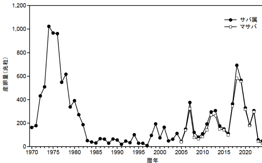
図 4-1. 本邦太平洋側におけるサバ属の産卵量 2005 年以降はマサバを分けて示した。2024 年は 1～6 月までの値。
