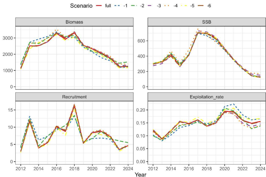
補足図 2-8. 各資源量指標値を除いたときの資源量等の推定値
