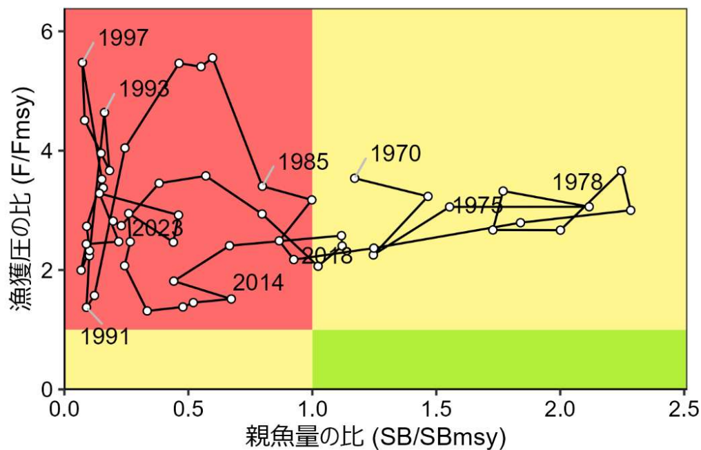
図 4-12. 最大持続生産量 (MSY) を実現する親魚量の代替値 (SBmsy proxy) と SBmsy proxy を維持する漁獲圧 (Fmsy proxy) に対する過去の親魚量および漁獲圧の関係 (神戸プロット)
