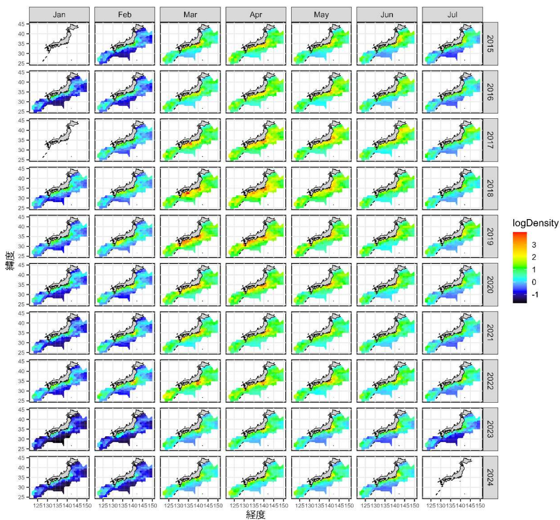
補足図 9-7b. 2015～2024 年（行）の 1～7 月（列）に推定されたマサバ卵密度 すべてのサンプルでマサバ卵が発見されなかった年・月の密度はゼロとした。
