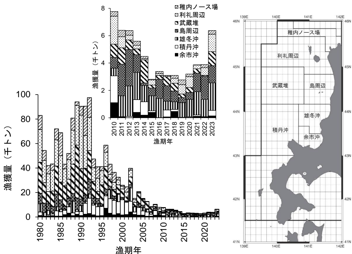
補足図 4-1. 北海道日本海側の沖底による小海区別のスケトウダラ漁獲量の推移 右上に 2010 年漁期以降の拡大図を示し、右の地図に各小海区の位置を示す。
