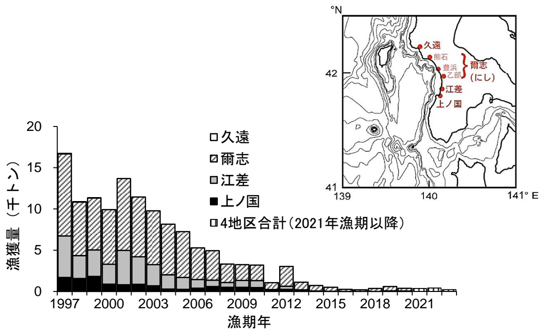
補足図 4-2. 檜山管内 4 地区における産卵親魚を対象とした延縄漁業（11 月～翌年 2 月）の漁獲量の推移 1997～2020 年漁期は地区別の漁獲量、2021 年漁期以降は 4 地区を合計した漁獲量を示す。（函館水産試験場 未発表資料）
