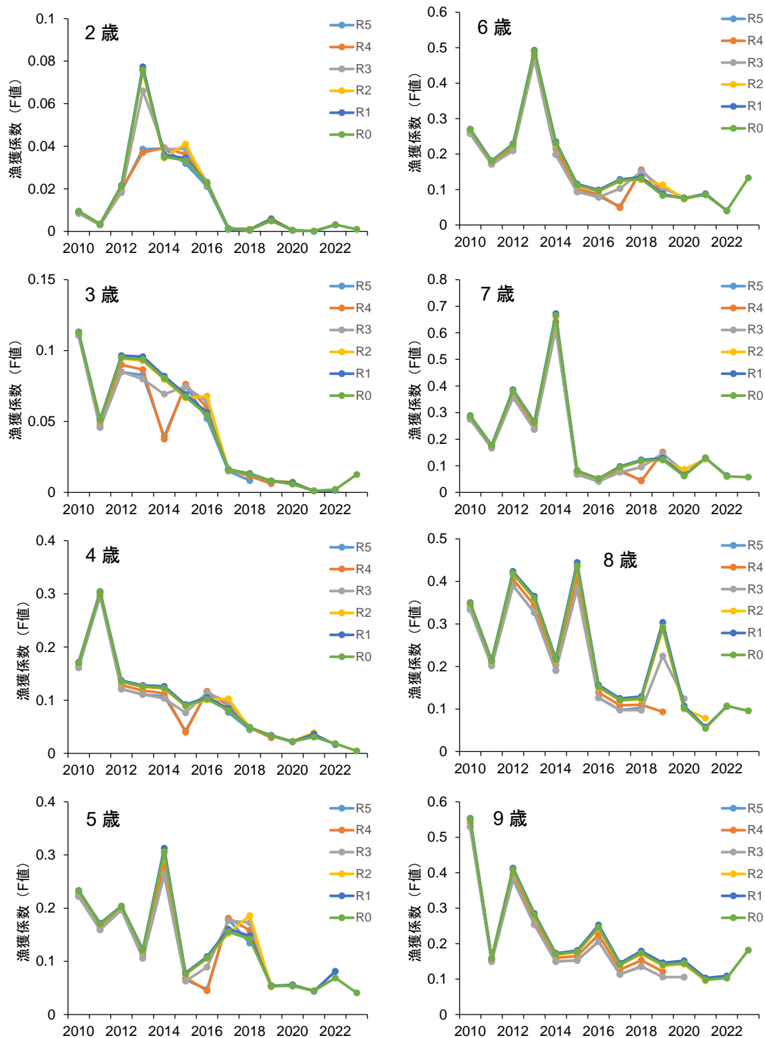
補足図 2-3b. レトロスペクティブ解析 ( \lambda=0.958 ) における各年齢の F の推移 R0 は最近年 (2023 年漁期) までのデータを用いた計算における推移、R1~R5 はそれぞれ 1~5 年分のレトロスペクティブ計算における推移を示す。
