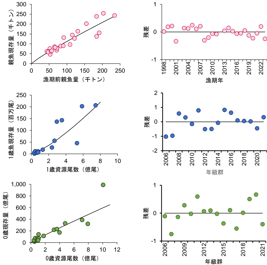
補足図 2-1. VPA で推定された親魚量や資源尾数と各調査の現存量推定値との関係 (左) および残差 (右)
