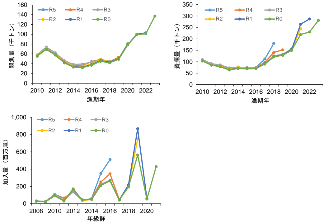
(b) \lambda=0.958 の場合
