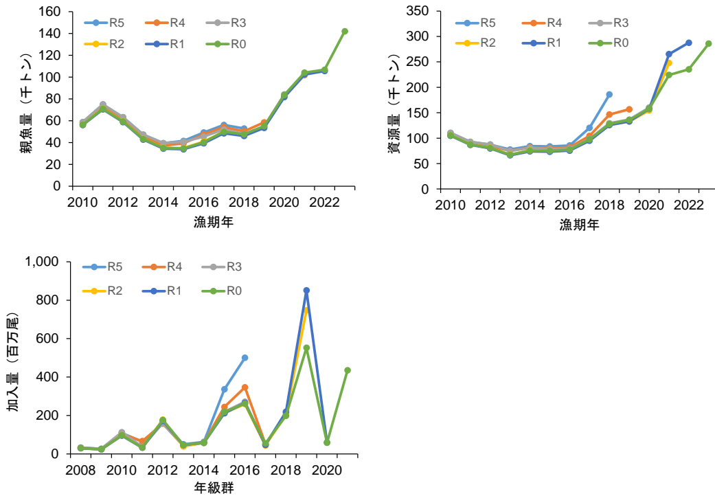
補足図 2-2. レトロスペクティブ解析における親魚量、資源量、加入量の推移
