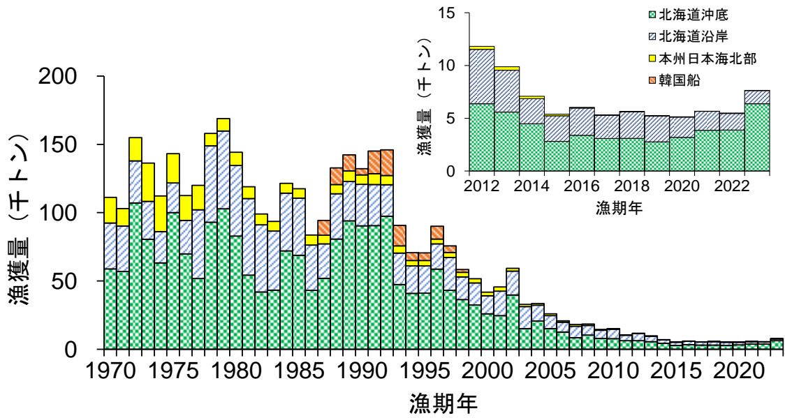
図 3-1. 漁獲量の推移 右上に 2012 年漁期以降を拡大した図を示す。
