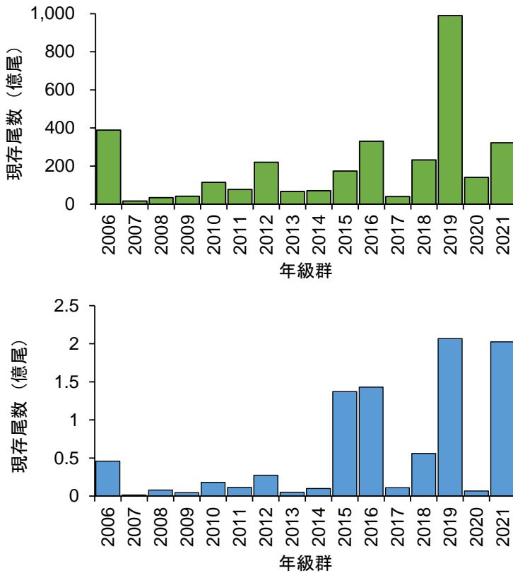
図 4-2. 加入量指標値の推移 上図は仔稚魚分布調査による0歳現存量推定値、下図は未成魚分布調査による1歳現存量推定値である（稚内・中央・函館水産試験場（印刷中）の図を改変）。
