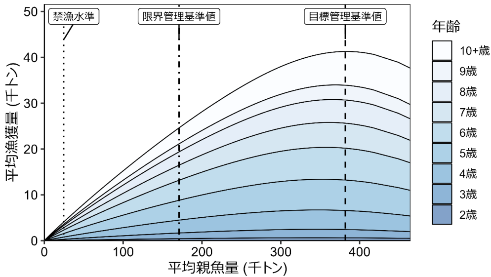
図 4-12. 平衡状態における平均親魚量と年齢別平均漁獲量の関係（千村ほか 2020）
