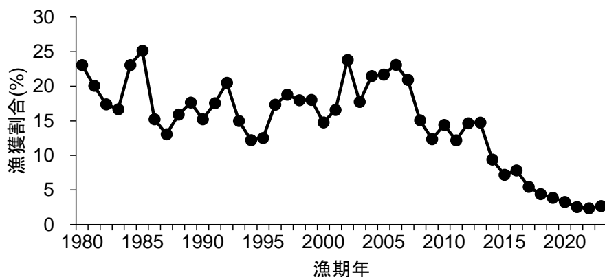
図 4-8. 漁獲割合の推移
