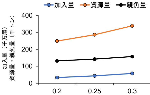
図 4-6. M の値を変化させた場合の 2023 年漁期の資源量、親魚量および加入量の変化 M は 3 歳以上の値を示す。2 歳の M はこの値に 0.05 を加算したものである。
