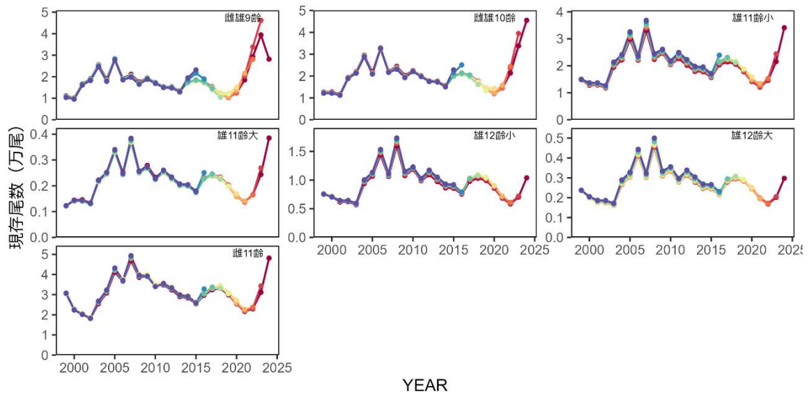
補足図 2-4. コホート解析のレトロスペクティブ分析結果 「小」は鋏脚小（未成熟・最終脱皮前）を、「大」は鋏脚大（成熟・最終脱皮後）を、それぞれ示す。
