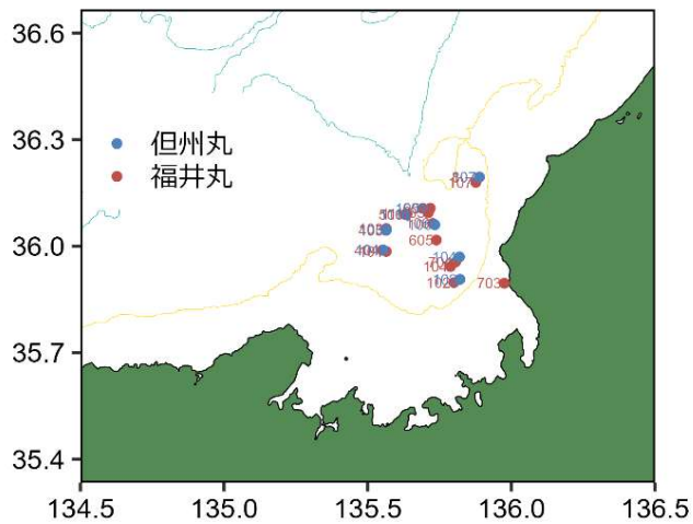
補足図 4-4. 隠岐西方（左図）および若狭沖（右図）での並行操業における調査点
