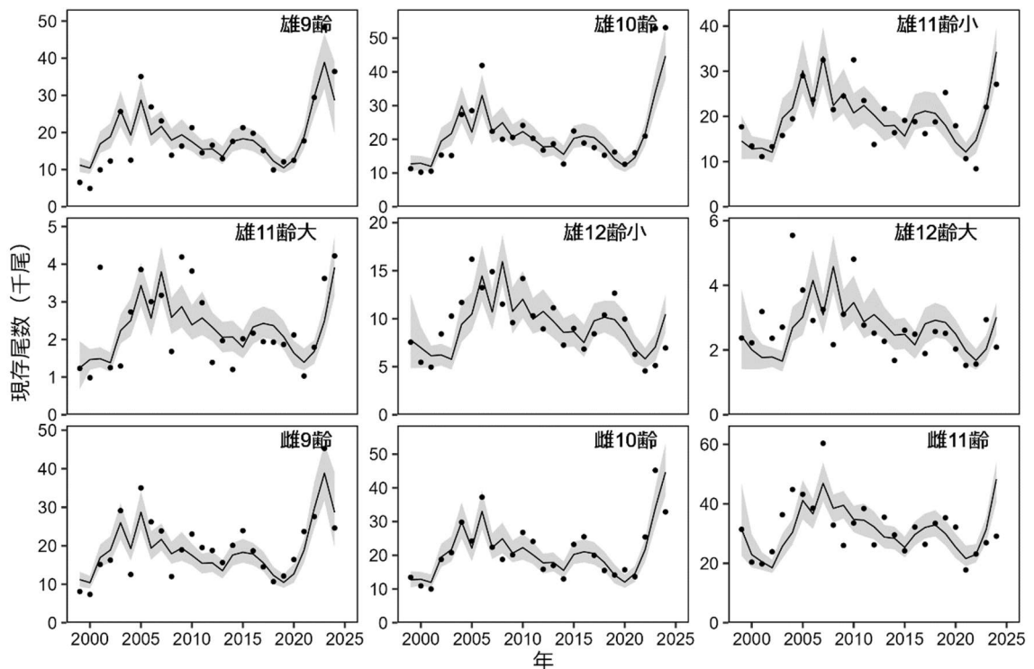
補足図 2-2. トロール調査による年別齢別現存尾数の観測値（黒点）および推定値（黒実線）
