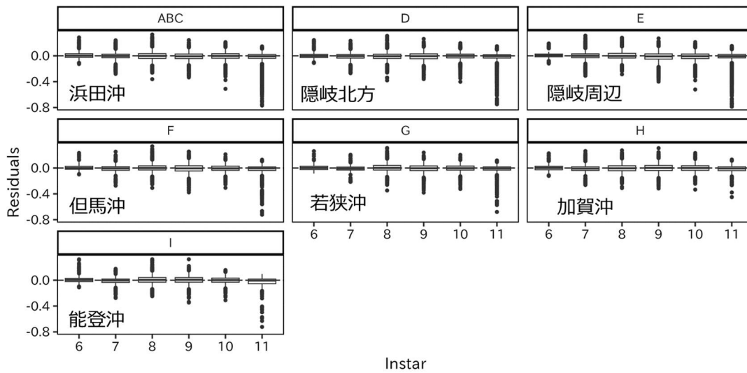
補足図 9-4. 当該モデルによる沖底小海区别齡期別の雌の逸脱度残差
