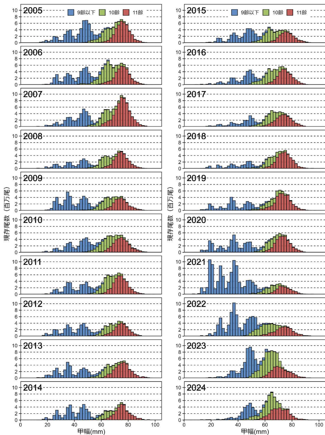
図 4-4. トロール調査から推定された近年の雌の甲幅組成 調査時点の 9、10、11 歳はそれぞれ、漁獲開始時点の未熟、アカコおよびクロコに相当する。
