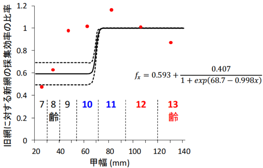
補足図 5-1. 並行調査および実際のトロール調査結果から推定された、旧網に対する新網の採集効率の比率 黒実線は並行調査による一般化ロジスティック式（右式）、赤丸は 2015 年の実際のトロール調査による齢期別の値をそれぞれ示す。
