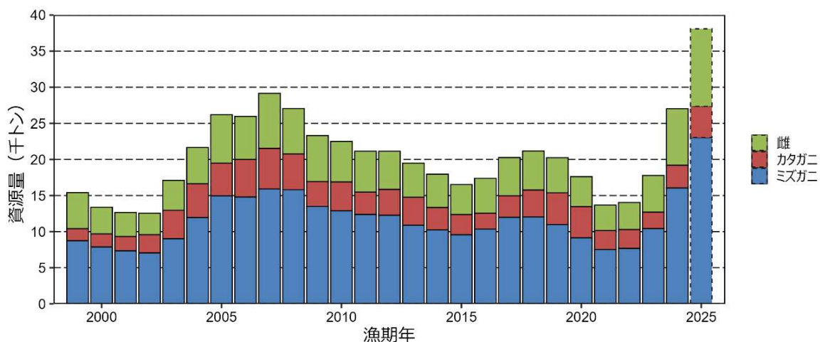
図 4-5. トロール調査結果に基づくコホート解析により推定された漁獲開始時点の資源量 ミズガニとカタガニは 12 歳と 13 歳の合計を、雌は 11 歳をそれぞれ示す。 2025 年は、2024 年の 10 歳以上の齢期別資源尾数等から前進計算により求めた予測値。
