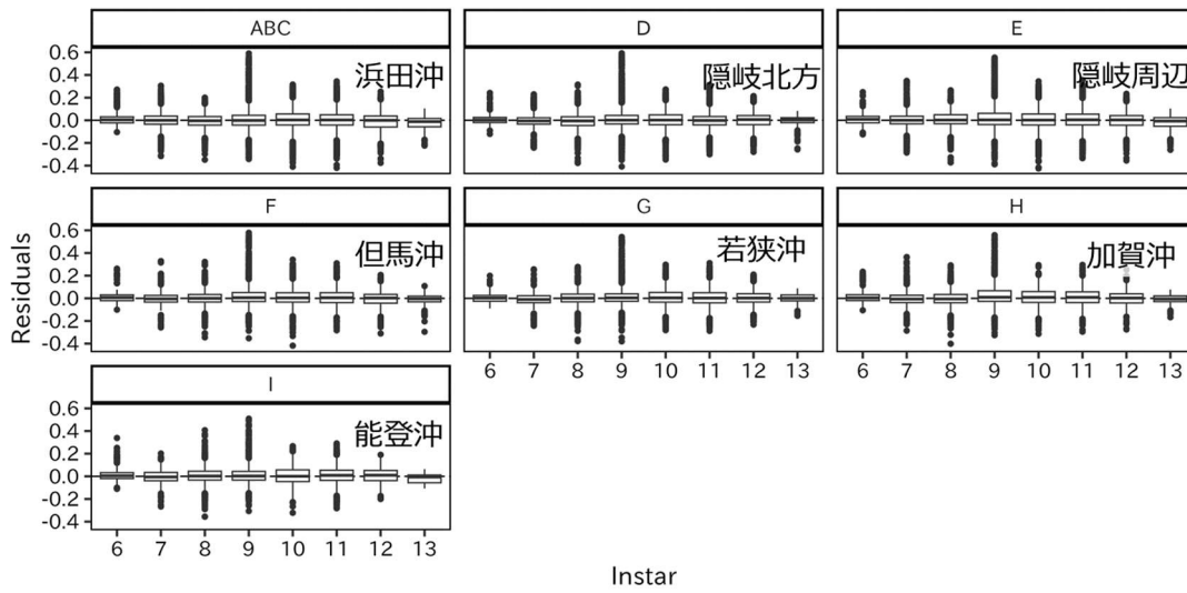
補足図 9-3. 当該モデルによる沖底小海区别齡期別の雄の逸脱度残差
