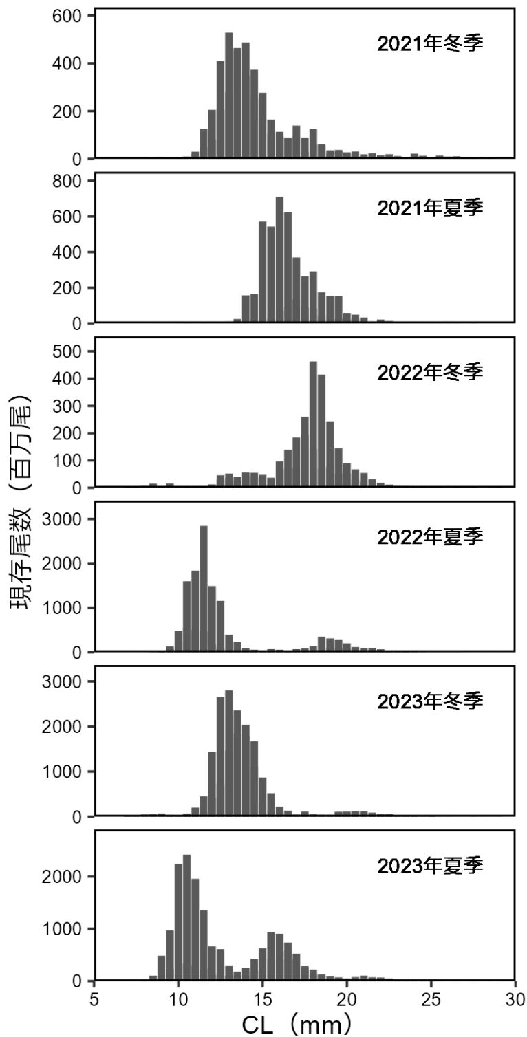
図 14. (続き) 石川県加賀沖においてソリ付き桁網調査で採集されたホッコクアカエビの頭胸甲長組成 2021~2023 年の冬季 (1~2 月) および夏季 (7~9 月) の調査結果に基づく水深 350~550 m における頭胸甲長階級 (0.5 mm) ごとの現存尾数。
