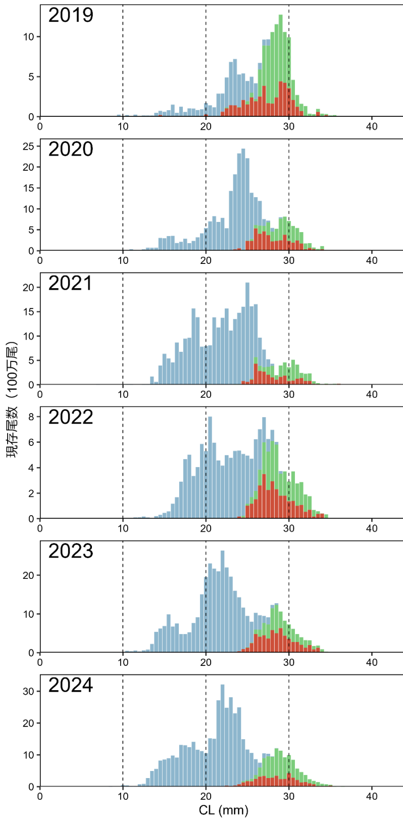
図 12. (続き) トロール調査に基づくホッコクアカエビの頭胸甲長組成 2019 年から 2024 年の若狭 (若狭沖、但馬沖に相当) における頭胸甲長階級 (0.5 mm) ごとの現存尾数を雄 (青)、抱卵雌 (赤)、非抱卵雌 (緑) 別に示した。
