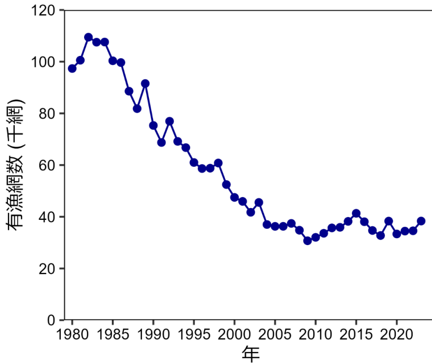
図 7. 沖底のホッコクアカエビ有漁網数
