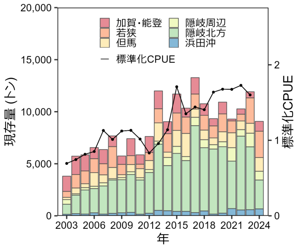
図 10. トロール調査に基づく日本海西部における現存量および沖底の標準化 CPUE 標準化 CPUE の値は平均値で除すことで、平均値が 1 になるよう規格化した。
