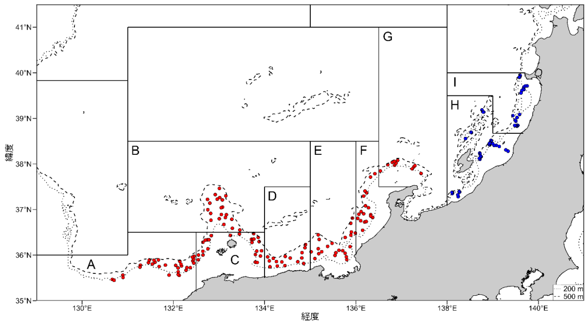
補足図 3-2. 本資料で使した沖底の小海区区分 A: 浜田沖 (従来の迎日南部 + 浜田沖); B: 隠岐北方; C: 隠岐周辺; D: 但馬沖; E: 若狭沖; F: 加賀沖; G: 能登沖; H: 新潟沖; I: 男鹿南部。赤丸はトロール調査、青丸は桁網調査の調査定点を示す。
