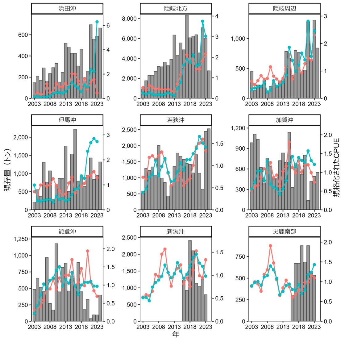
補足図 3-3. 小海区別沖底標準化 CPUE (赤線)、ノミナル CPUE (青線) および現存量 (棒グラフ) の推移。両 CPUE は比較のため全年の平均が 1 となるように平均値で除すことで規格化している。現存量はトロール調査 (浜田沖～能登沖) および桁網調査 (新潟沖および男鹿南部) に基づく面積密度法により推定した。
