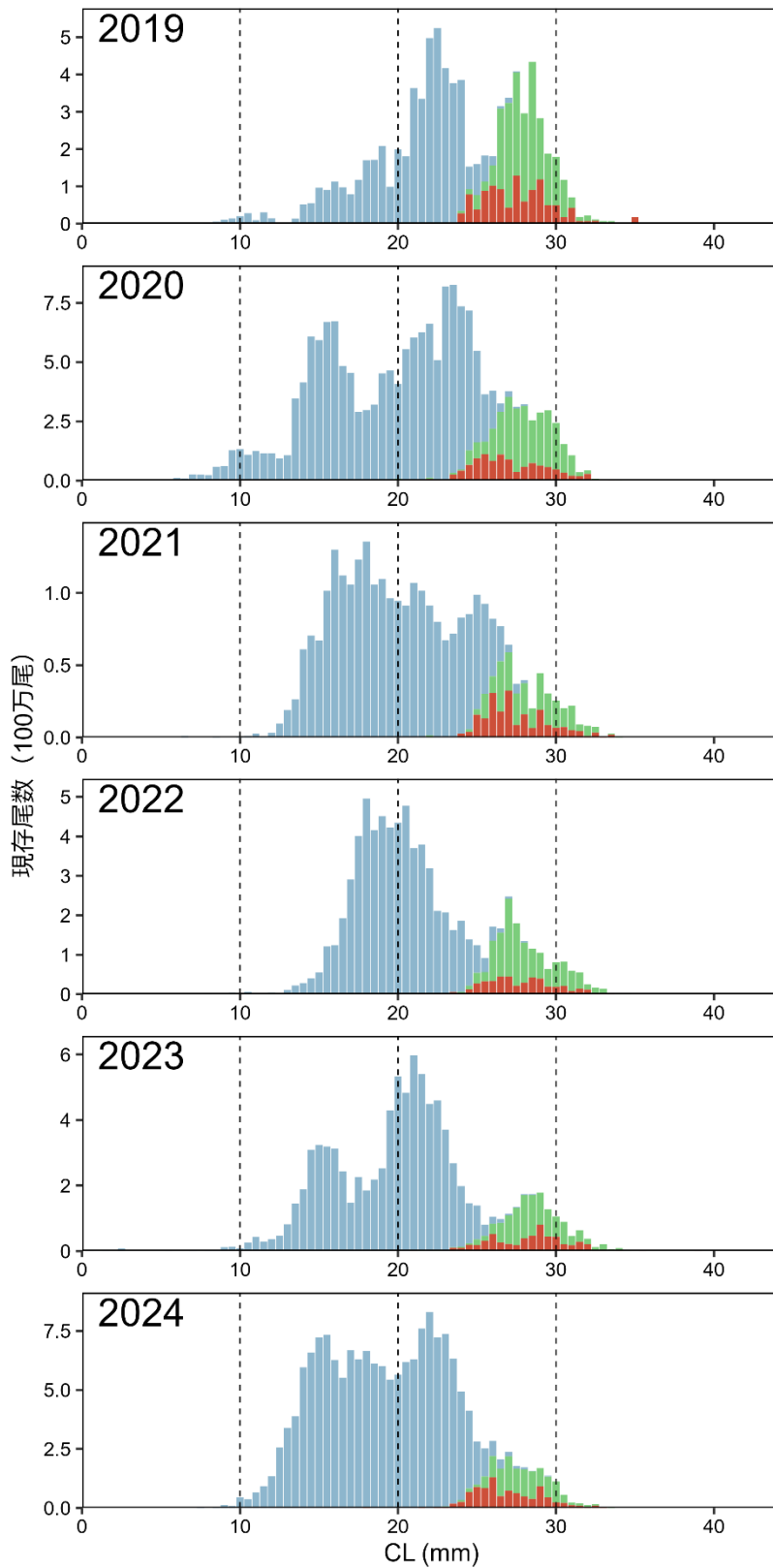
図 12. (続き) トロール調査に基づくホッコクアカエビの頭胸甲長組成 2019 年から 2024 年の能登（能登沖、加賀沖に相当）における頭胸甲長階級（0.5 mm）ごとの現存尾数を雄（青）、抱卵雌（赤）、非抱卵雌（緑）別に示した。
