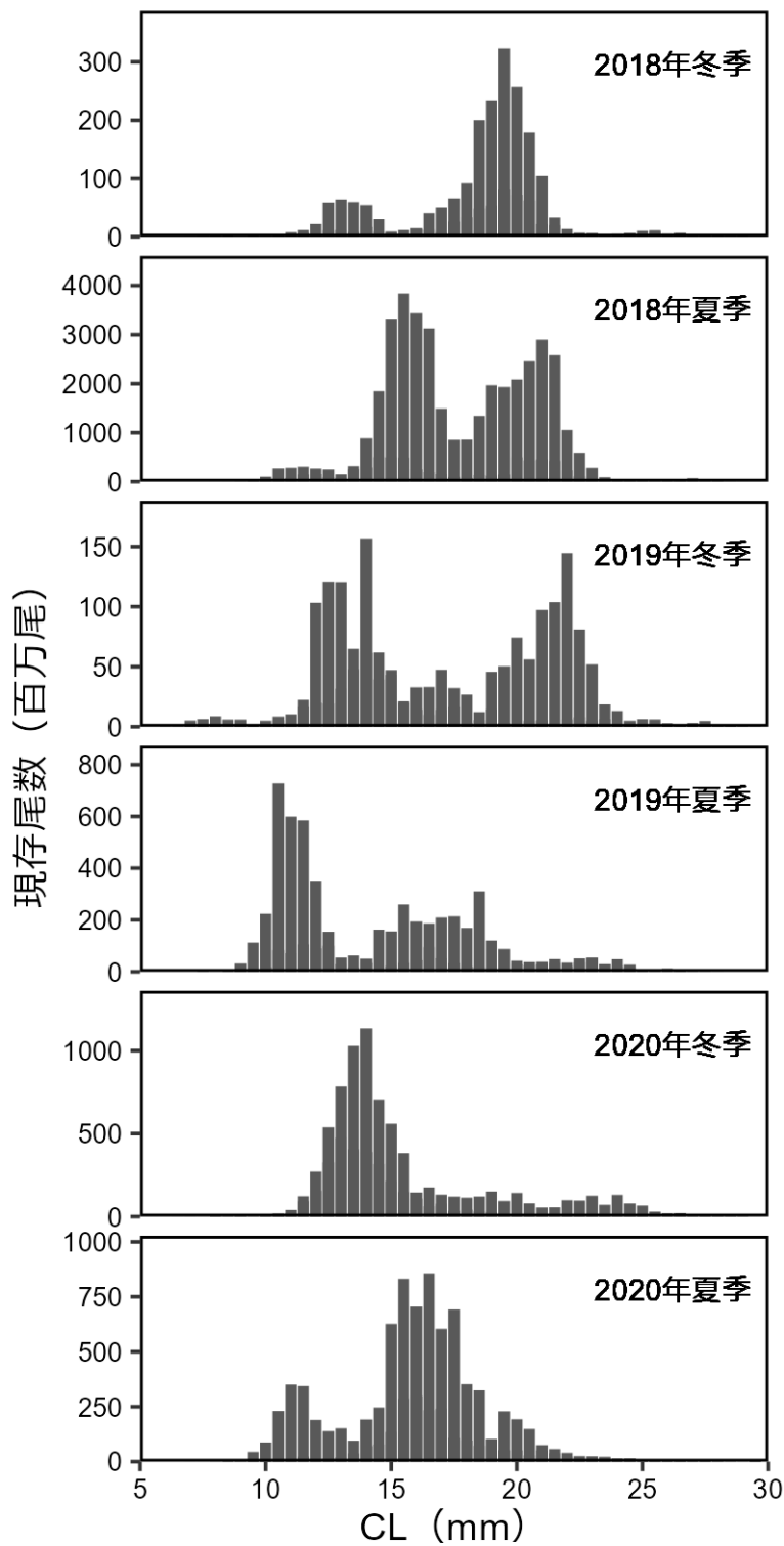
図 14. 石川県加賀沖においてソリ付き桁網調査で採集されたホッコクアカエビの頭胸甲長組成 2018～2020 年の冬季（1～2 月）および夏季（7～9 月）の調査結果に基づく水深 350～550 m における頭胸甲長階級（0.5 mm）ごとの現存尾数。
