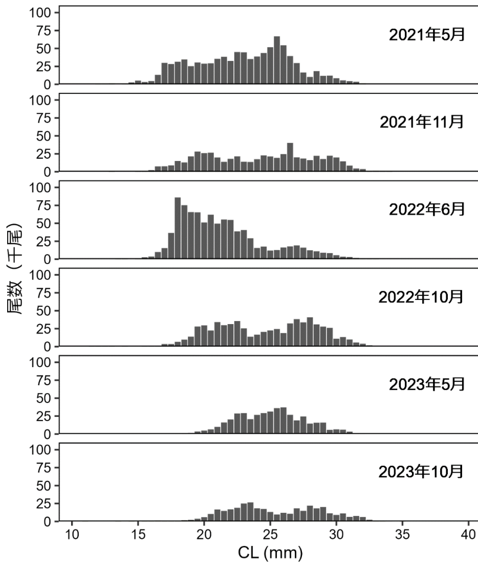
図 13. 金沢港（石川県）における漁獲物の頭胸甲長組成 各調査日における 1 隻 1 日分の銘柄別組成および全船の水揚げ箱数から、当日の頭胸甲長階級（0.5 mm）ごとの総水揚げ尾数を推定した。
