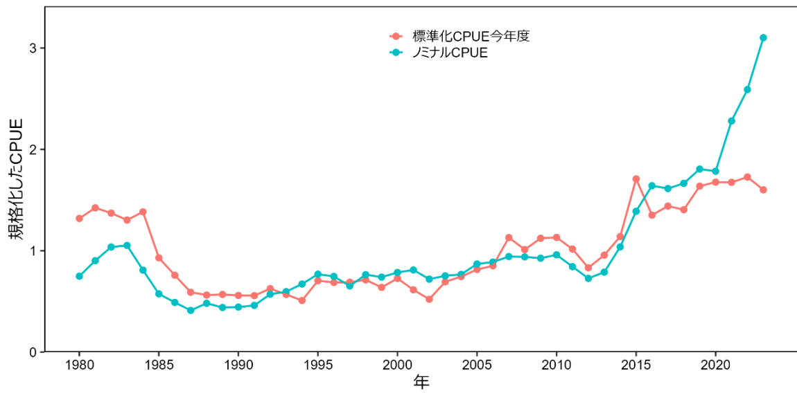
補足図 2-1. 標準化 CPUE およびノミナル CPUE の推移 比較のため全年の平均が 1 となるように平均値で除すことで規格化している。
