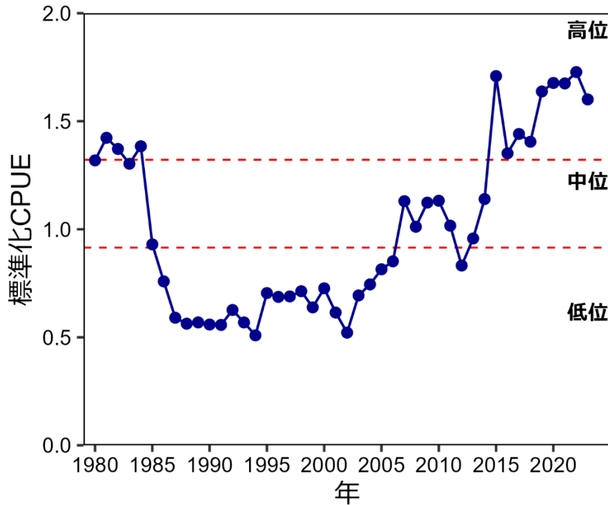
図 8. 沖底の標準化 CPUE の推移、および資源水準の区分 標準化 CPUE の値は平均値で除すことで、平均値が 1 になるよう規格化した。
