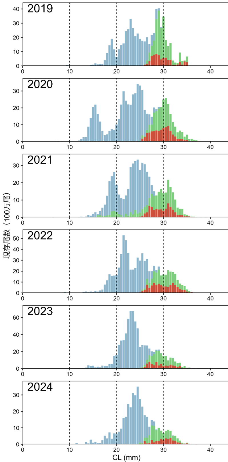
図 12. トロール調査に基づくホッコクアカエビの頭胸甲長組成 2019 年から 2024 年の 隠岐（沖底小海区の浜田沖、隠岐北方、隠岐周辺に相当）における頭胸甲長階級 (0.5 mm) ごとの現存尾数を雄（青）、抱卵雌（赤）、非抱卵雌（緑）別に示した。
