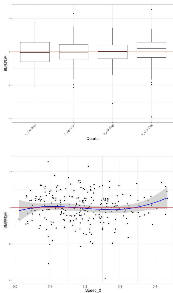
図 6. ベストモデルの層別逸脱残差 Speed_0に関する残差図の青線と灰帯は、残差にフィッティングさせた平滑化曲線（loess）と、その 95%信頼区間を示す。
