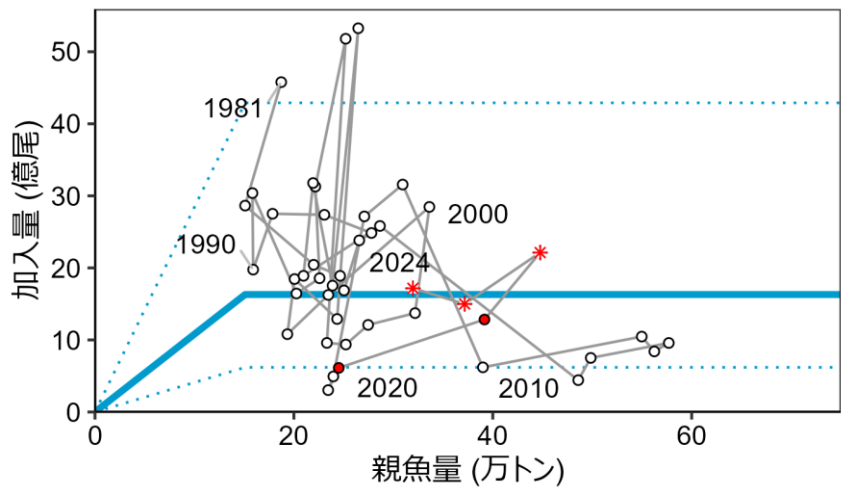
図7 再生産関係
