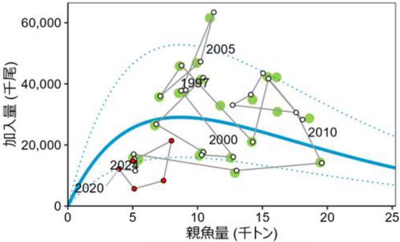
図6 再生産関係
