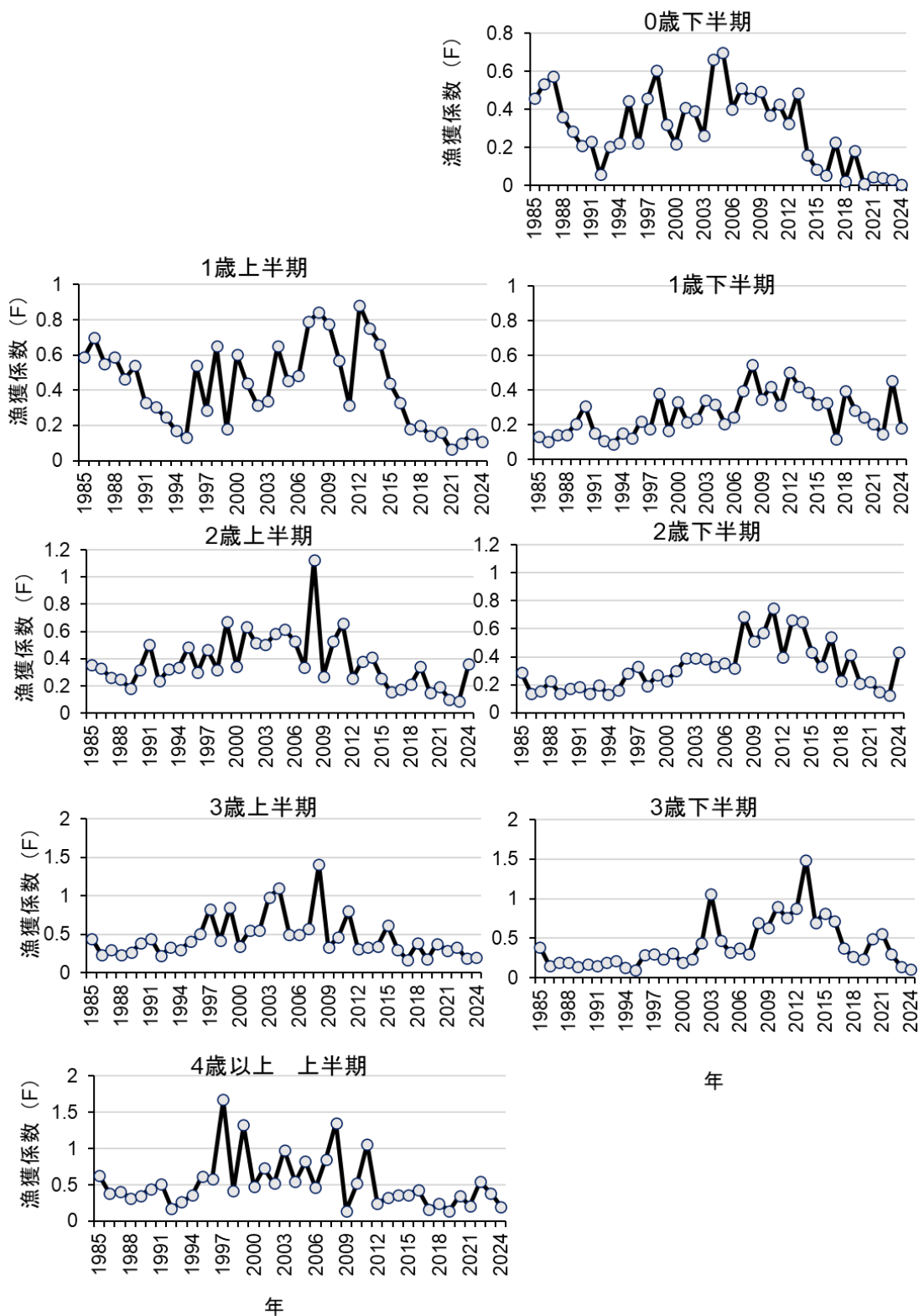
図 4-6. 各年齢の半期別 F 値の経年推移
