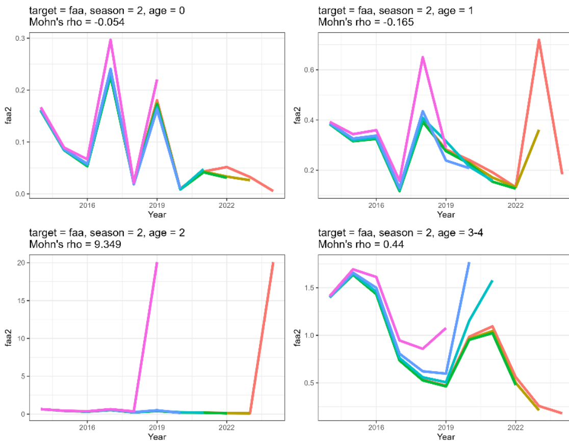
補足図 12-4b. 今年度採用した沖底 CPUE および昨年度と同じ指数間の重みを用いた場合の下半期における年齢別Fのレトロスペクティブ解析結果(指数間の重みを沖底CPUE: 1歳 CPUE = 8.2 : 1.8 とし、リッジペナルティは使用していない)
