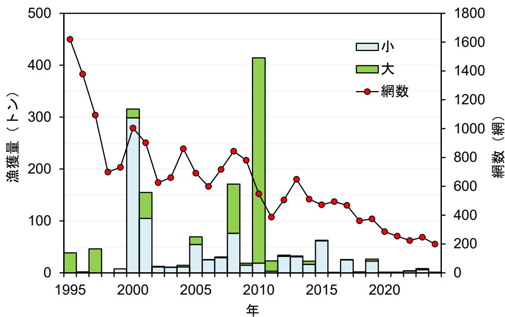
図 3-4. 日本海中部および北部（東経 135.5 度以东）における大中型まき網のサワラ漁獲 量（小：1.6 kg 以下、大：1.6 kg 以上）と網数
