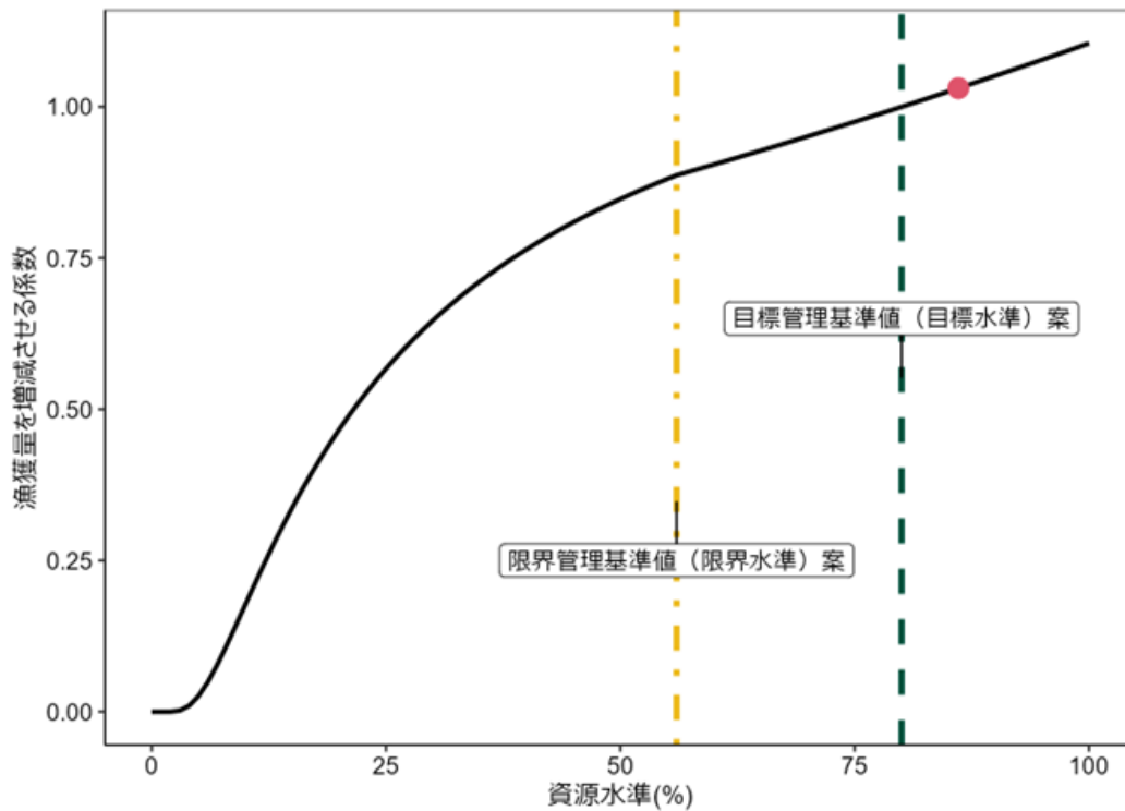
補足図 3-2. 漁獲管理規則案
