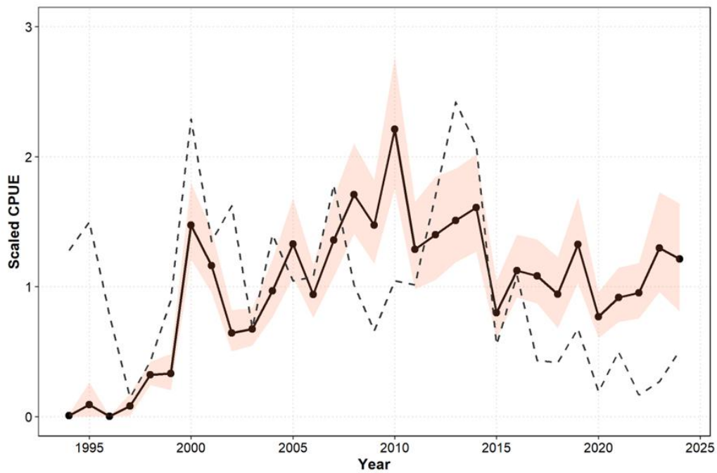
補足図 2-1. 大中型まき網により漁獲されたサワラの平均値で規格化した 95%信頼区間付き標準化 CPUE (赤) およびノミナル CPUE (破線)
