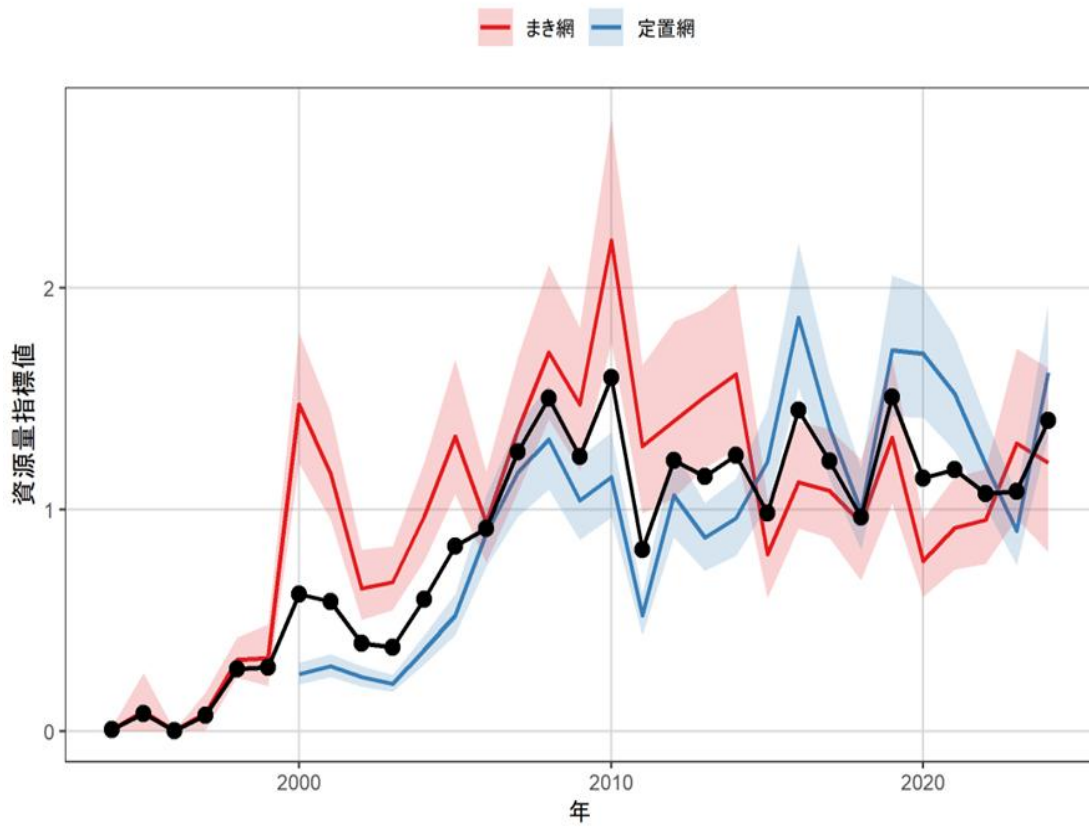
図 4-1. 資源量指標値の推移（赤は大中型まき網の標準化 CPUE、青は定置網の標準化 CPUE、黒が資源量指標値となるそれらの相乗平均値）
