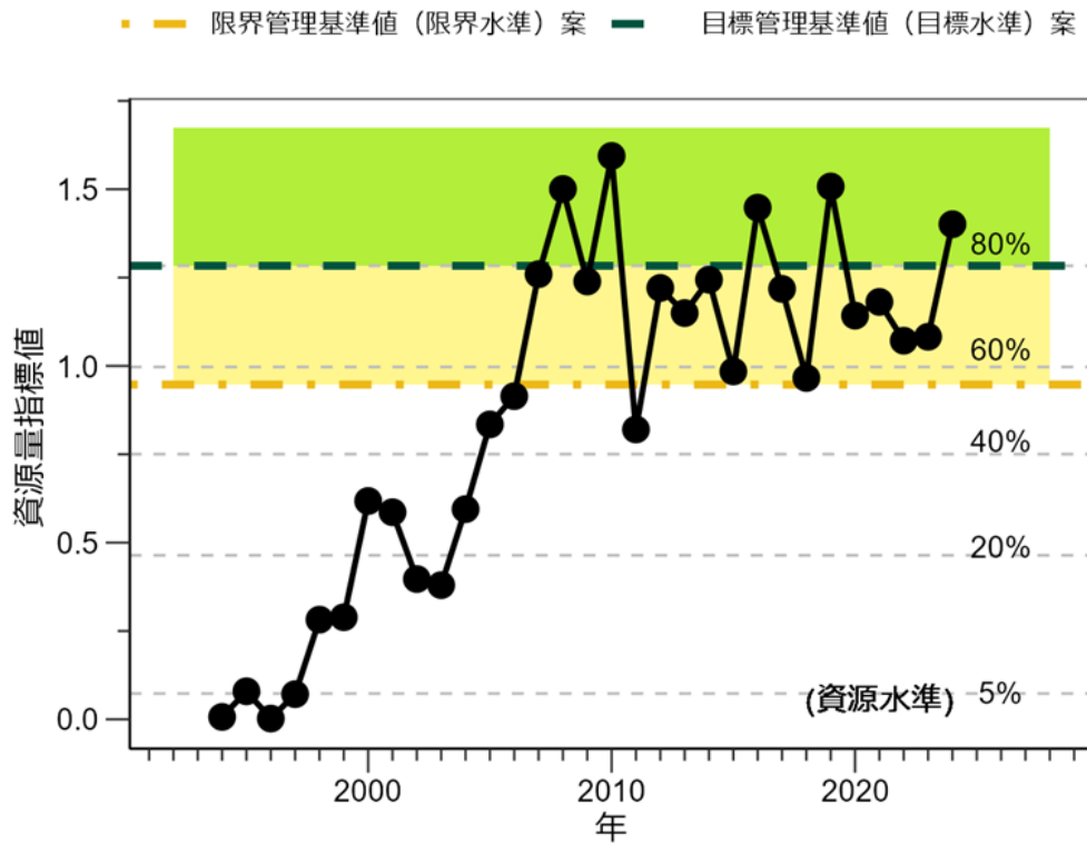
補足図 3-1. 資源量指標値の推移と目標水準案、限界水準案
