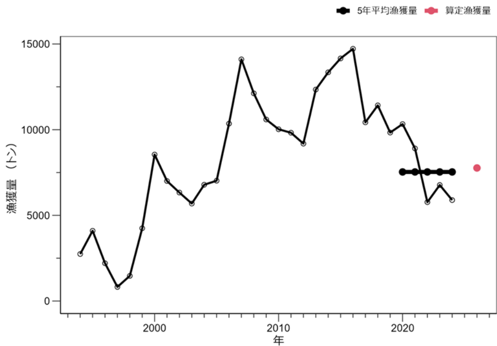
補足図 3-3. 漁獲量の推移と試算された直近 5 年平均の漁獲量および算定漁獲量
