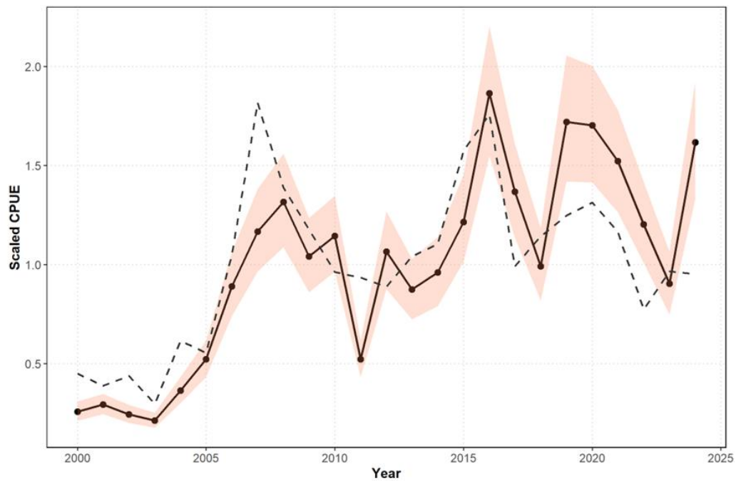
補足図 2-2. 定置網により漁獲されたサワラの平均値で規格化した 95%信頼区間付き標準化 CPUE (赤) およびノミナル CPUE (破線)
