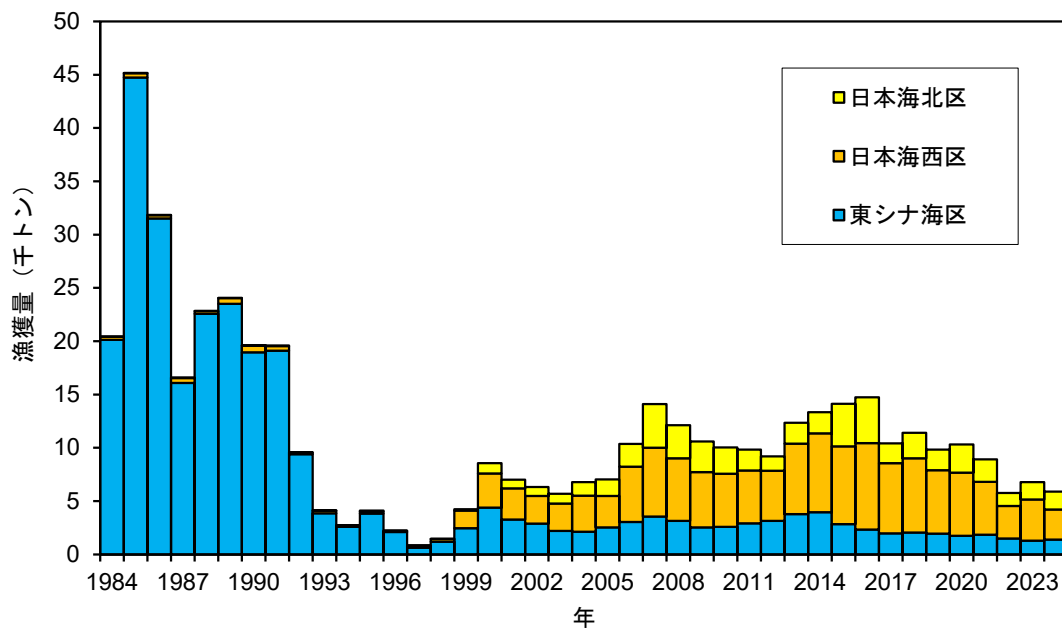
図 3-1. 日本漁船による海區別漁獲量（日本海北区：青森県～石川県、日本海西区：福井県～山口県、東シナ海区：福岡県～鹿児島県）
