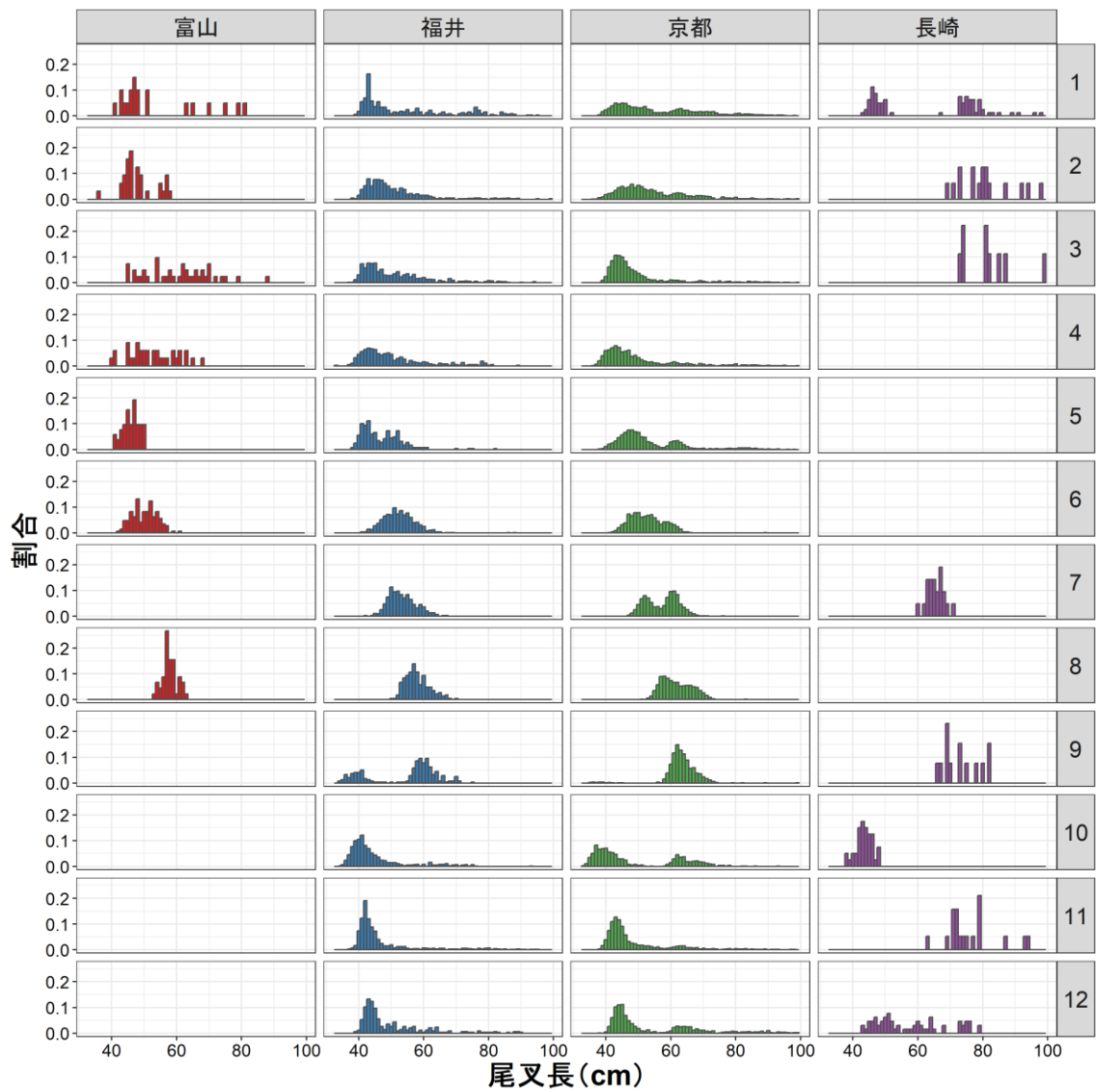
図 4-4. 新潟県、富山県、福井県、京都府、長崎県におけるサワラの 2024 年月別尾叉長組成
