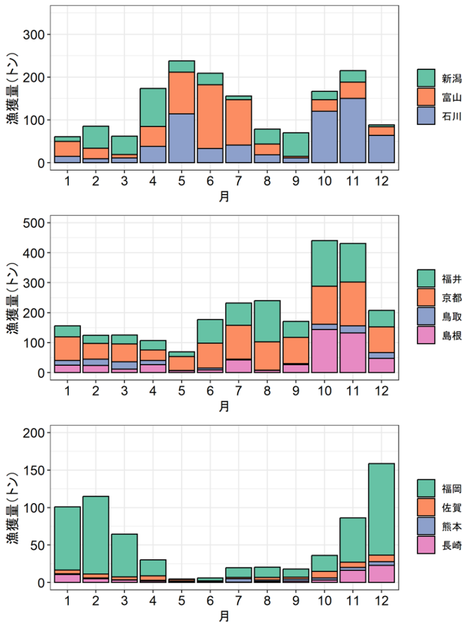
図 3-2. 2024 年における海区別 (上：日本海北区 (新潟県、富山県、石川県)、中：日本海西区 (福井県、京都府、鳥取県、島根県)、下：東シナ海区 (福岡県、佐賀県、長崎県、熊本県)) 月別漁獲量
