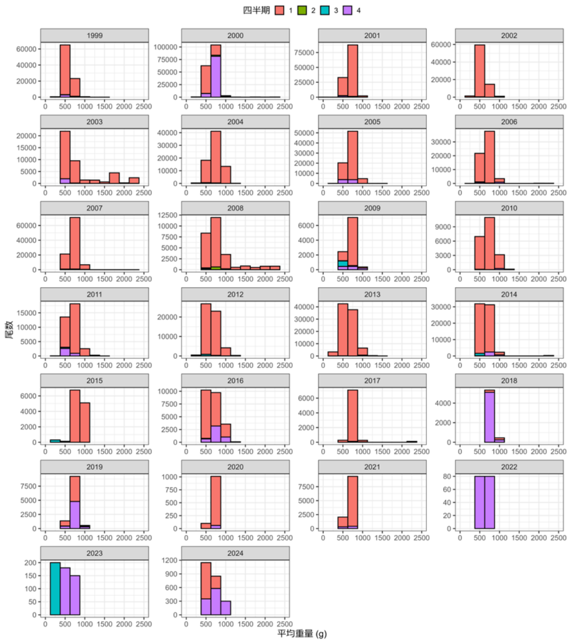
図 4-3. 大中型まき網により九州主要港に水揚げされたサワラの体重別漁獲尾数（第 1 四半期：1～3 月、第 2 四半期：4～6 月、第 3 四半期：7～9 月、第 4 四半期：10～12 月）
