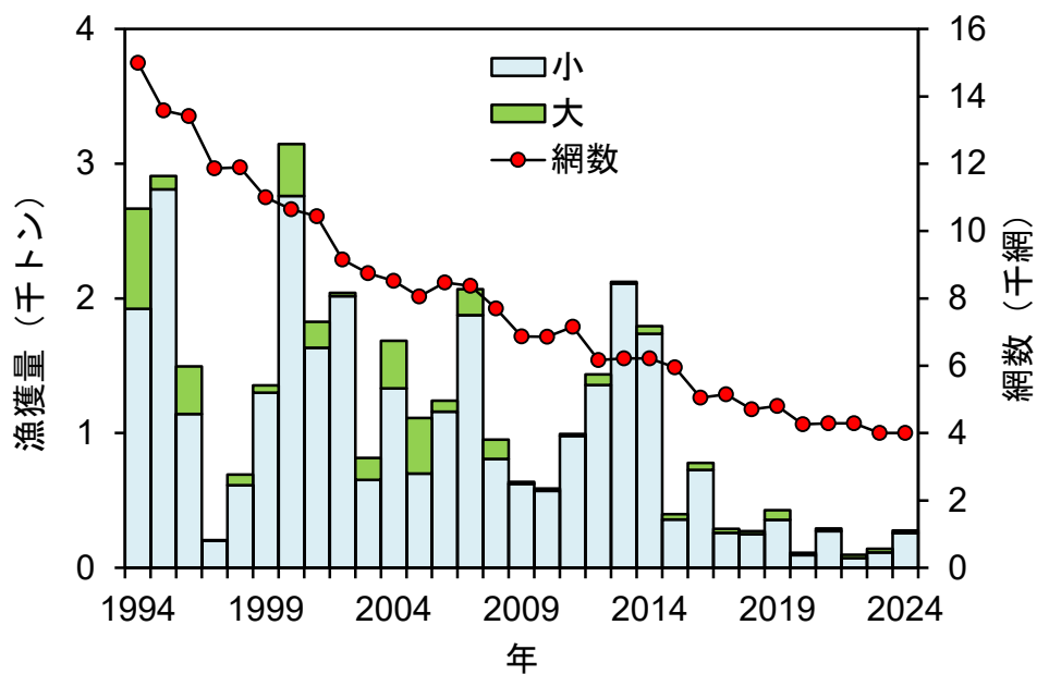
図 3-3. 日本海西部（東経 135.5 度以西）および東シナ海における大中型まき網のサワラ 銘柄別漁獲量（小：1.6 kg 以下、大：1.6 kg 以上）と網数
