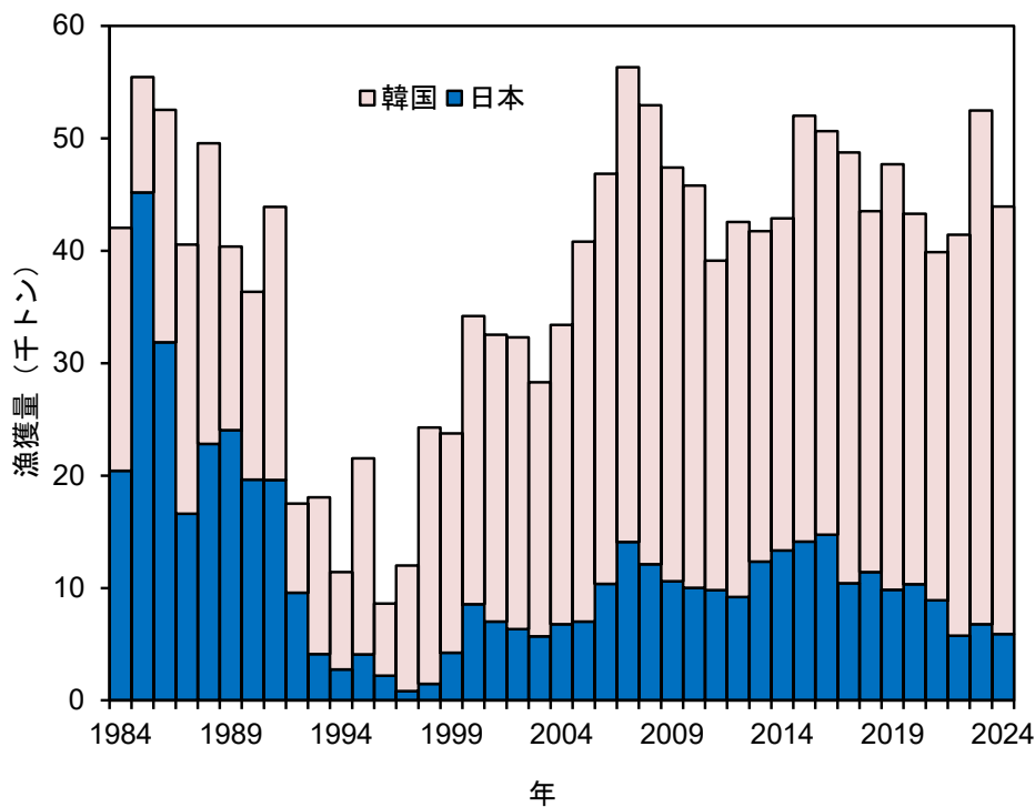
図 3-6. 日本および韓国の漁獲量
