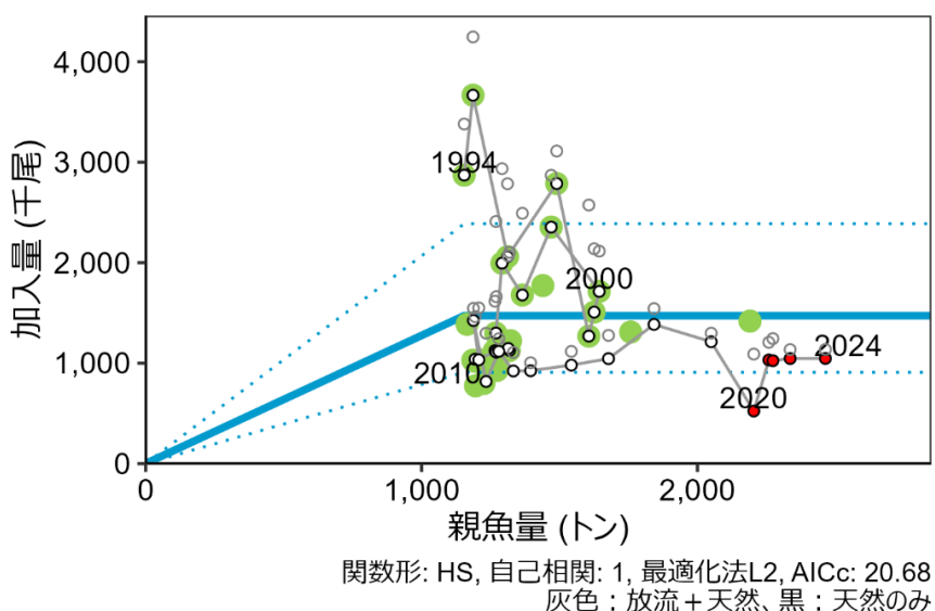
図 4-12. 親魚量と加入量の関係（再生産関係）
