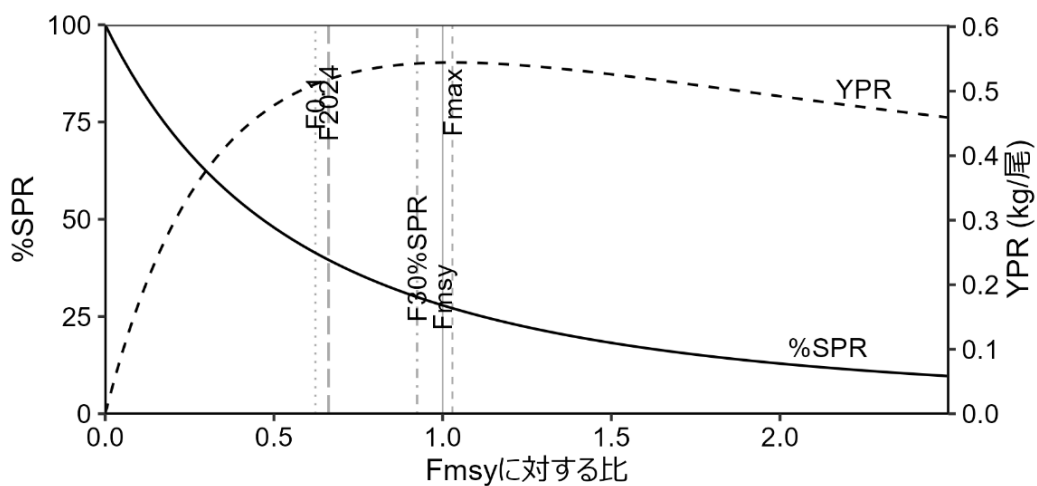
図 4-11. Fmsy に対する YPR、%SPR の関係
