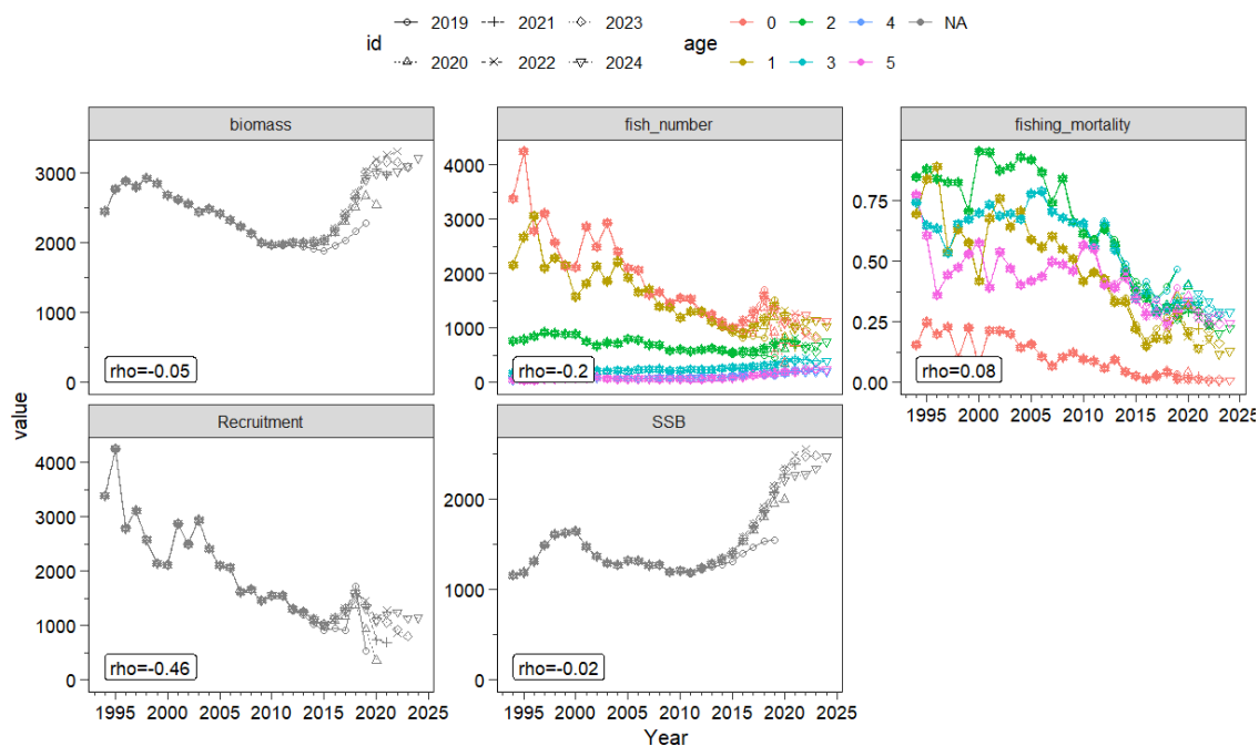
補足図 2-2. 資源量 (biomass、トン)、資源尾数 (fish number、千尾)、漁獲係数 (fishing_mortality)、0 歳資源尾数 (Recruitment、千尾)、親魚量 (SSB、トン) のレトロスペクティブ解析結果
