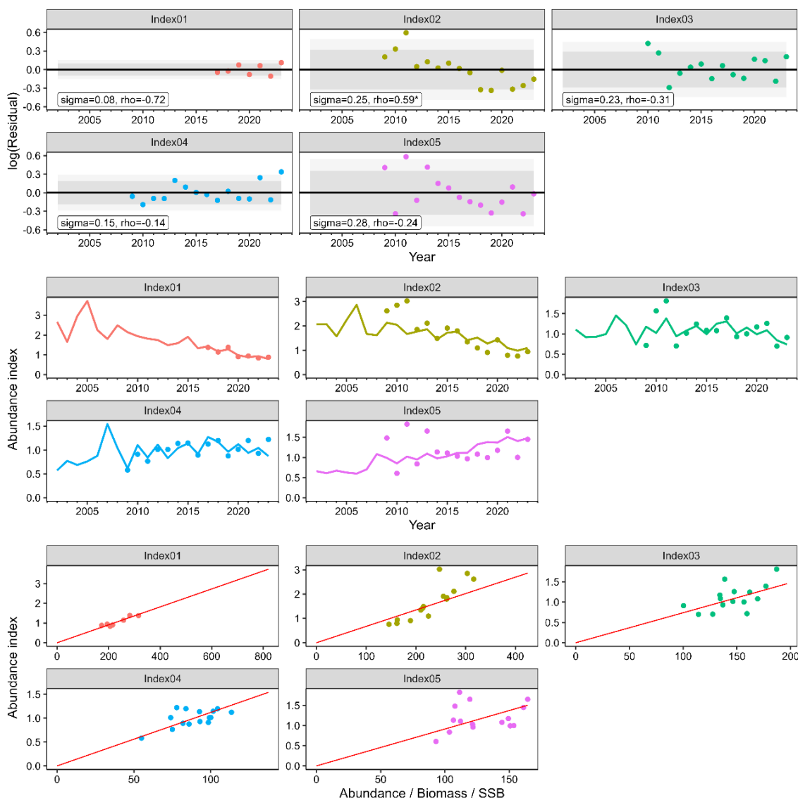
資料図 10-5. 検討 1 (最尤法、 b 推定なし) における残差プロット、指標値 (○) と予測値 (実線)、各年齢の指標値と年齢別資源尾数との相関。残差プロットのダークグレーは 80%信頼区間、ライトグレーは 95%信頼区間を示す。対数残差には、尤度 ( \sigma : sigma)、Mohn's rho ( \rho ) を示した。 \rho のアスタリスクは自己相関係数が有意に大きい場合を示す。Index01 : 0 歳 CPUE、Index02 : 1 歳 CPUE、Index03 : 2 歳 CPUE、Index04 : 3 歳 CPUE、Index05 : 4 歳以上 CPUE。
