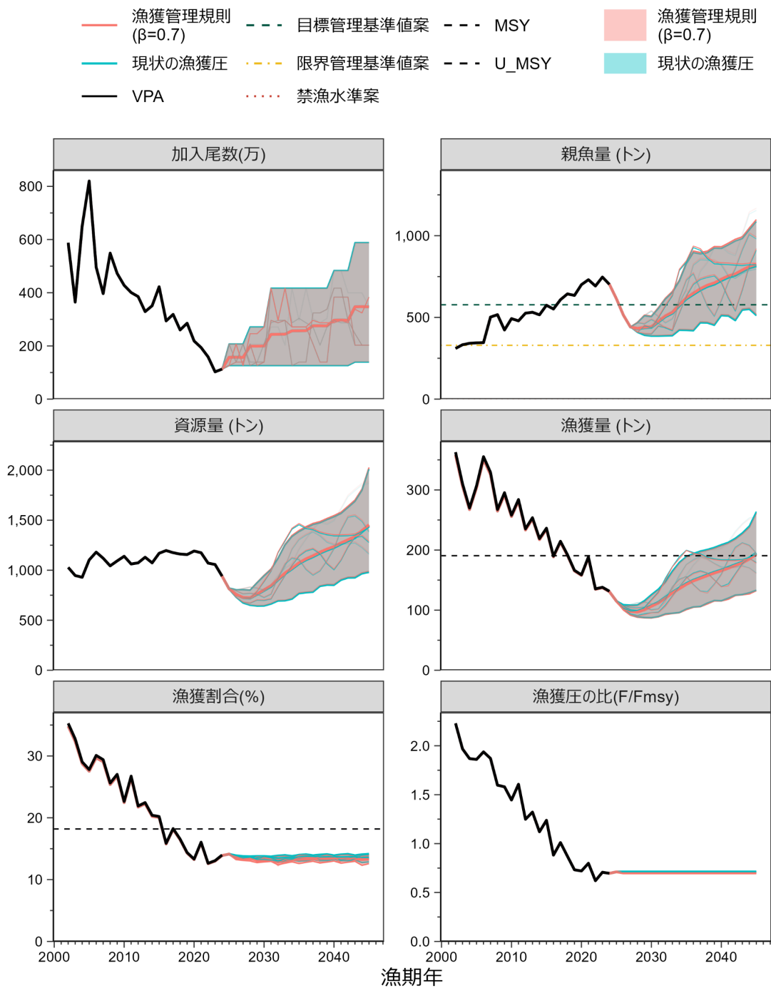
補足図 7-6. 漁獲管理規則案を用いた場合（赤線）と現状の漁獲圧での将来予測（青色） （2025 年漁期以降は、2016～2020 年漁期の平均放流加入尾数を仮定（仮定 4）） 太 実線は平均値、網掛けはシミュレーション結果の 90%が含まれる予測区間、細線は 5 通りの将来予測の例示である。親魚量の図の緑破線は目標管理基準値案、黄一点鎖線 は限界管理基準値案、赤点線は禁漁水準案を示す。漁獲割合の図の破線は U_{msy} を示 す。漁獲管理規則での調整係数 \beta には 0.7 を用いた。
