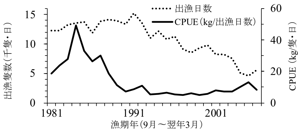
図 3-16. 山口県瀬戸内海側のはえ縄の努力量と単純 CPUE の推移
