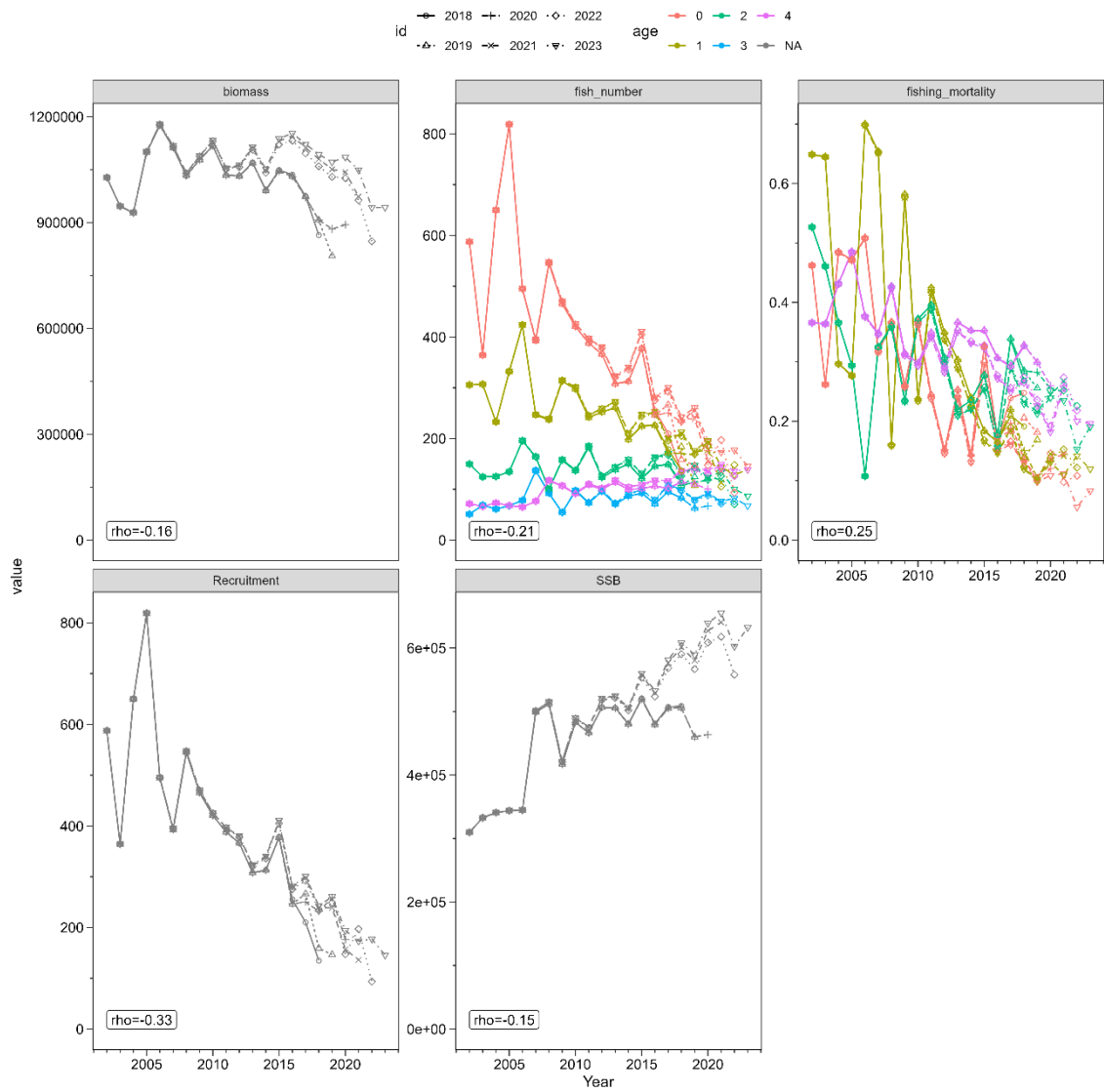
資料図 10-12. 検討3 (最小二乗法、b 推定なし) におけるレトロスペクティブ解析の結果
