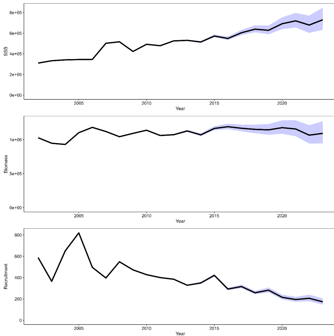
資料図 10-14. 検討 1 (最尤法、 b 推定なし) におけるブートストラップ信頼区間推定結果 紫色の影の範囲は 95%信頼区間を示す。上から順に、親魚量 (単位: トン)、資源量 (単位: トン)、0 歳資源尾数 (単位: 千尾)。
