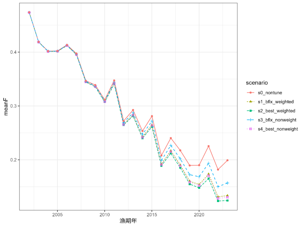
資料図 10-4. 試算結果の比較 (F平均) S0 : チューニングなし。S1 : 検討1、S2 : 検討2、S3 : 検討3、S4 : 検討4。各検討の条件は補足表 10-1 を参照。
