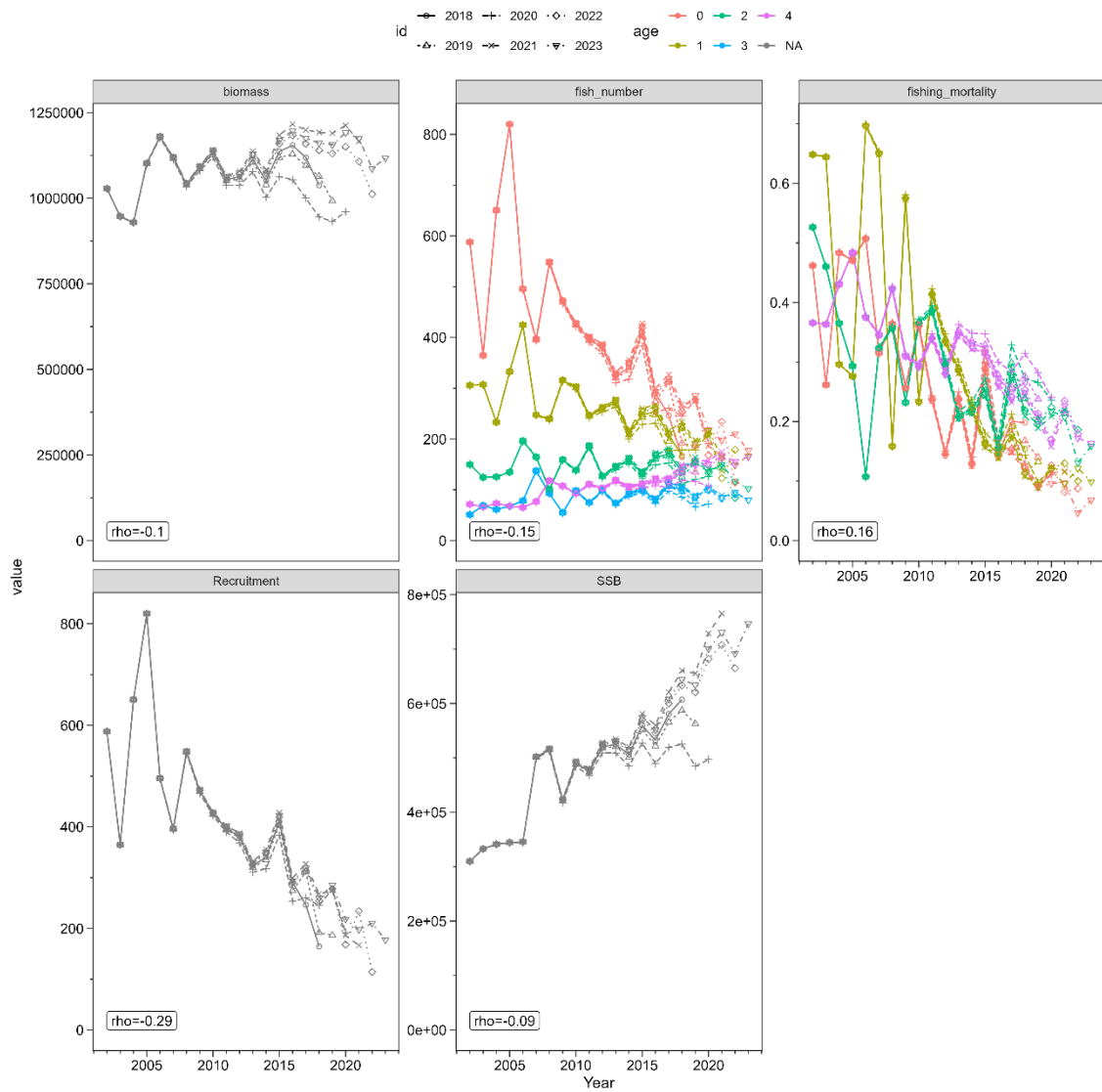
資料図 10-13. 検討 4 (最小二乗法、b 推定あり) におけるレトロスペクティブ解析の結果
