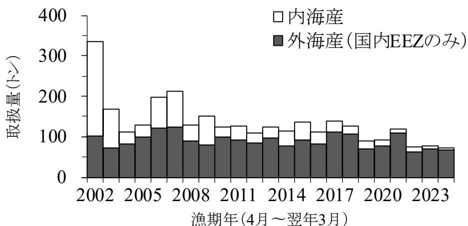
図 3-1. 下関唐戸魚市場の取扱量の推移（上段：資料全期間、下段：本系群資源評価期間） 2020年漁期以前は、同市場の内海産、外海産銘柄に基づく。2021年漁期以降は、同市場の府県別取扱量に基づき、本系群の日本海・東シナ海産（有明海、八代海を含む）を外海産、それ以外を内海産として扱った。
