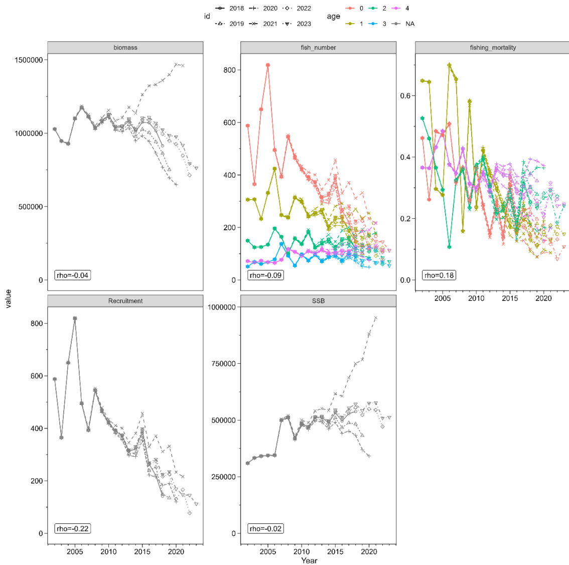
資料図 10-9. チューニングなしの VPA におけるレトロスペクティブ解析の結果
