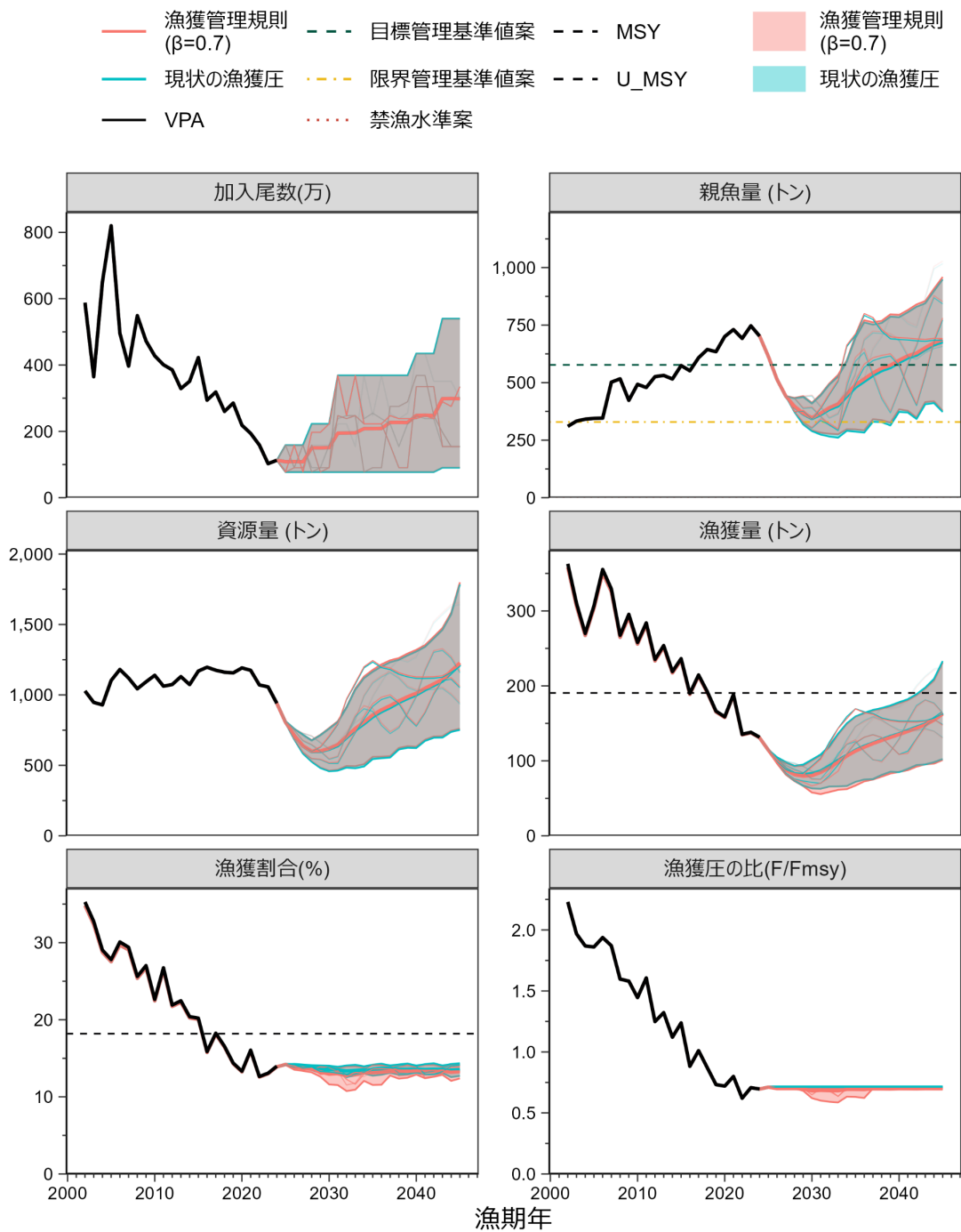
補足図 7-8. 漁獲管理規則案を用いた場合（赤線）と現状の漁獲圧での将来予測（青色） （2025 年漁期以降は、2024 年漁期の平均放流加入尾数を仮定（仮定 6））太実線は 平均値、網掛けはシミュレーション結果の 90%が含まれる予測区間、細線は 5 通りの 将来予測の例示である。親魚量の図の緑破線は目標管理基準値案、黄一点鎖線は限界 管理基準値案、赤点線は禁漁水準案を示す。漁獲割合の図の破線は U_{msy} を示す。漁 獲管理規則での調整係数 \beta には 0.7 を用いた。
