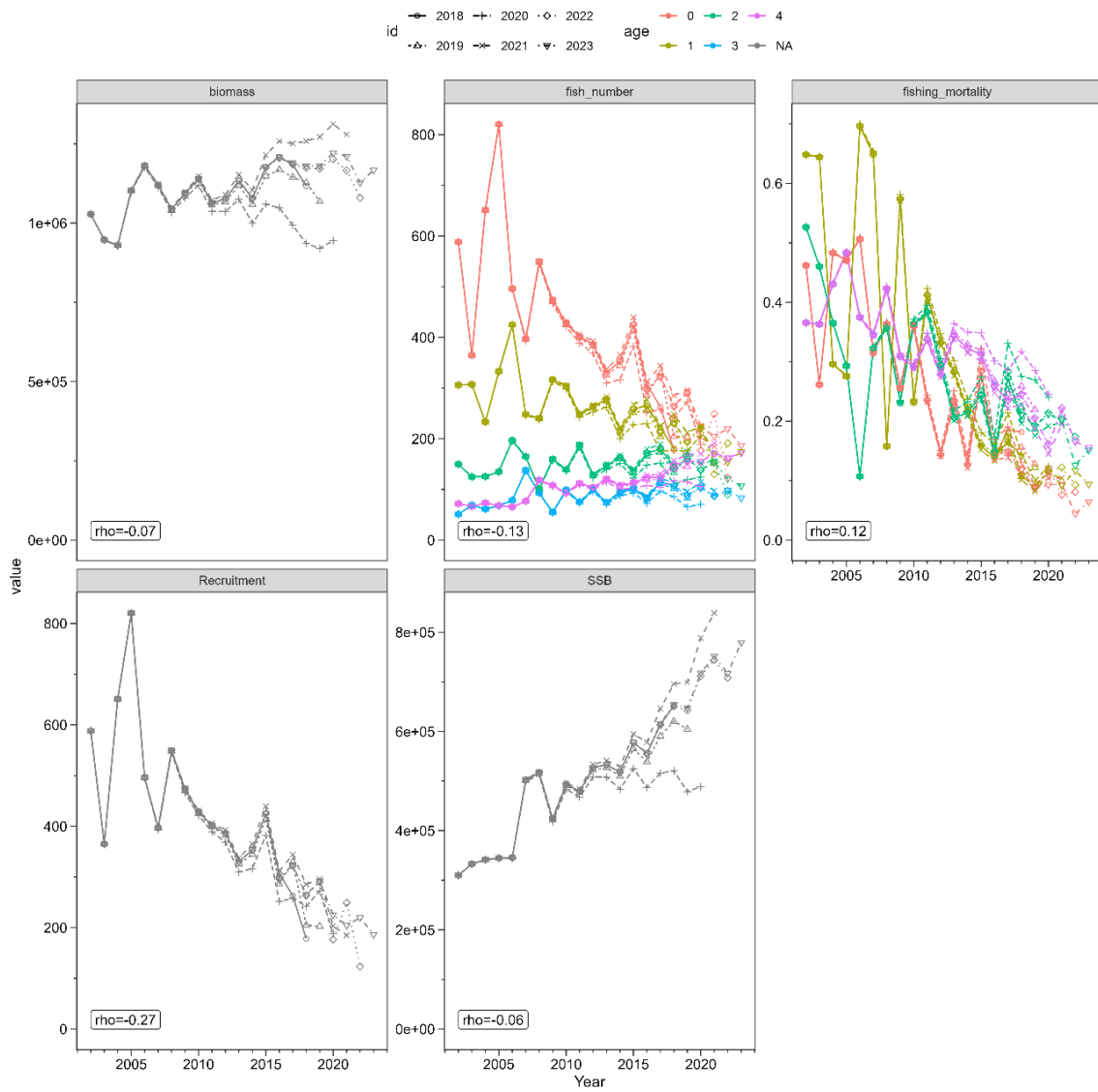
資料図 10-11. 検討 2 (最尤法、b 推定あり) におけるレトロスペクティブ解析の結果
