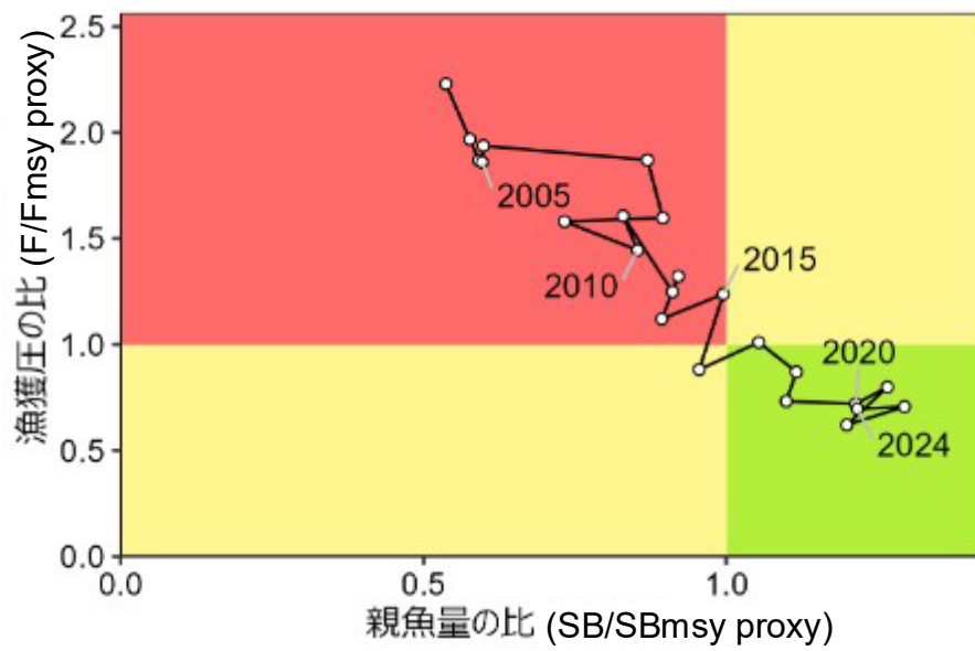
図 4-9. 最大持続生産量 (MSY) を実現する親魚量の代替値 (SBmsy proxy) と MSY を実現する漁獲圧の代替値 (Fmsy proxy) に対する過去の親魚量および漁獲圧の関係 (神戸プロット)
