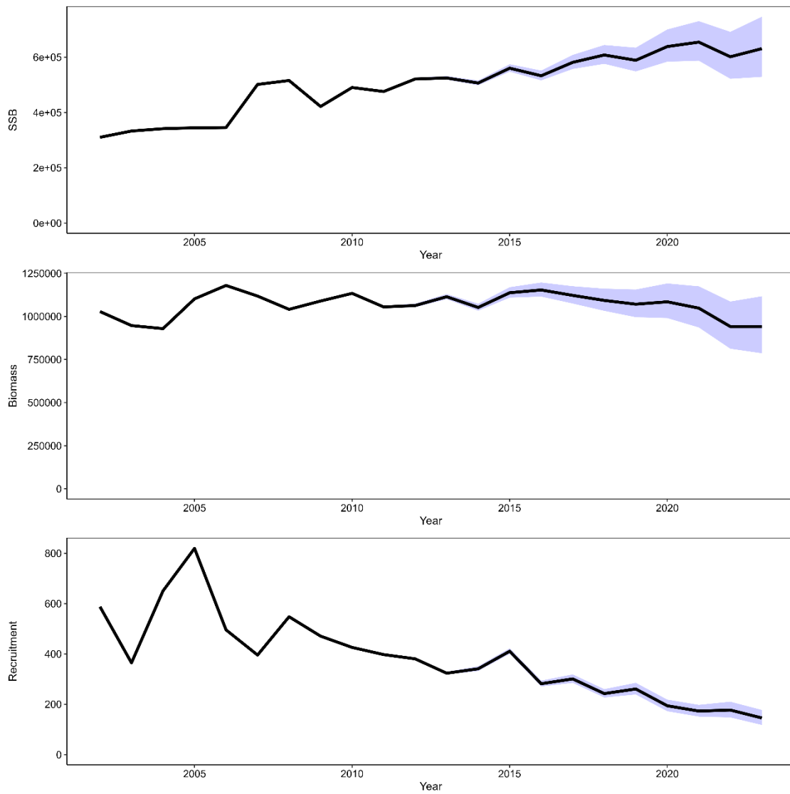
資料図 10-16. 検討 3 (最小二乗法、b 推定なし) におけるブートストラップ信頼区間推定結果 紫色の影の範囲は 95%信頼区間を示す。上から順に、親魚量 (単位: トン)、資源量 (単位: トン)、0 歳資源尾数 (単位: 千尾)。
