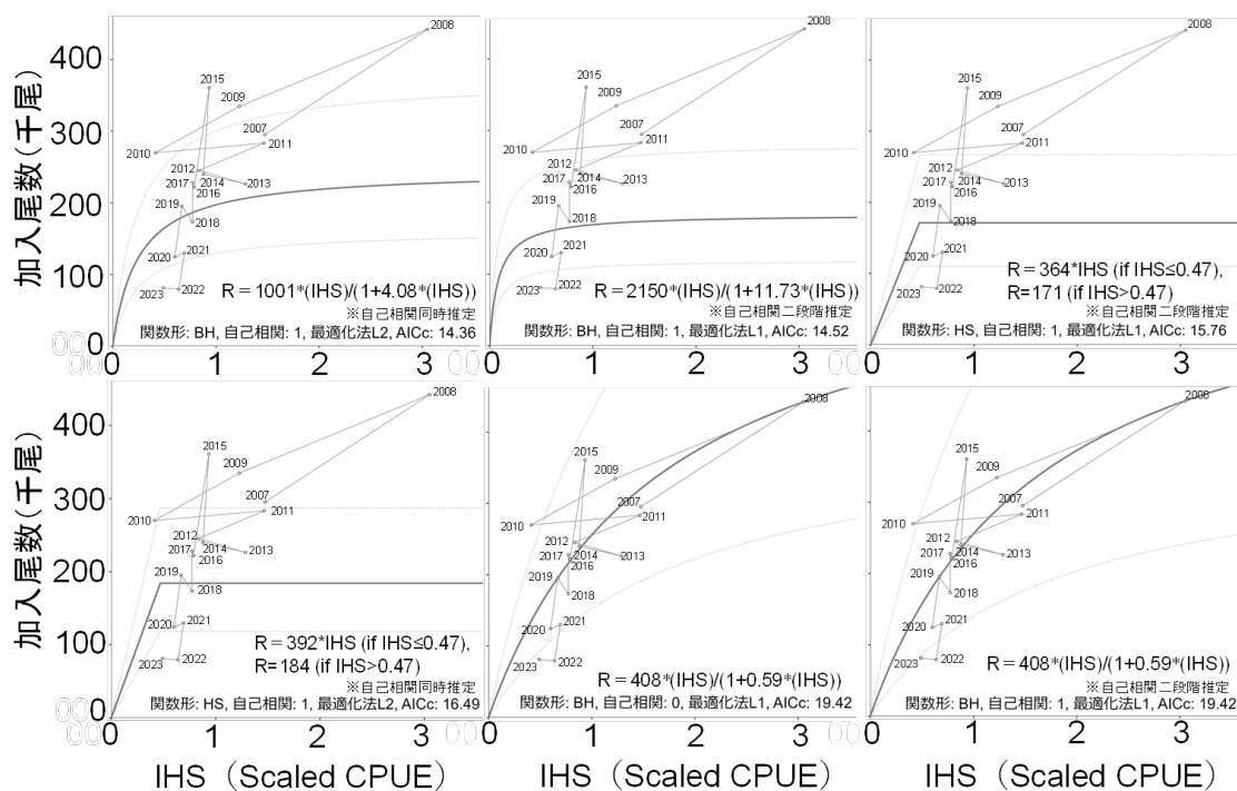
補足図 10-3. 再生産関係式に基づく産卵来遊指標値 (IHS) と 0 歳天然資源尾数との関係 AICc が最小から順に上位 6 モデルの比較結果。
