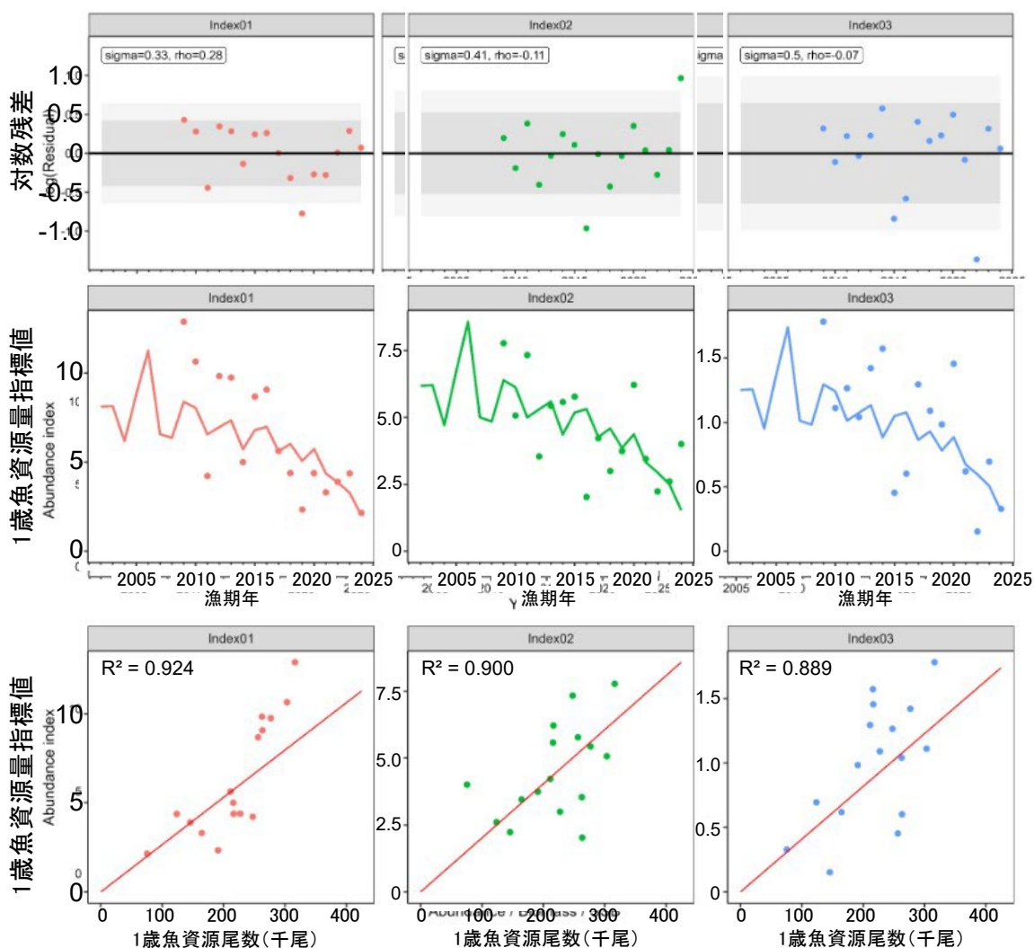
補足図 4-5. 1 歳魚資源量指標値のモデル診断
