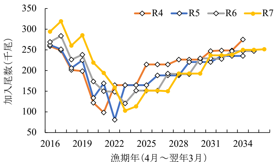
補足図 7-2. 3年ブロックのバックワード・リサンプリングに基づく将来予測における加入尾数の予測結果 (A) 天然のみによる加入を仮定した場合(仮定3)。(B) 放流込みでの加入を仮定した場合(仮定5)。放流尾数については直近5年の2019～2023年漁期の平均放流資源尾数を適用。天然のみの場合は、2025年漁期のみを放流考慮した場合を示す。
