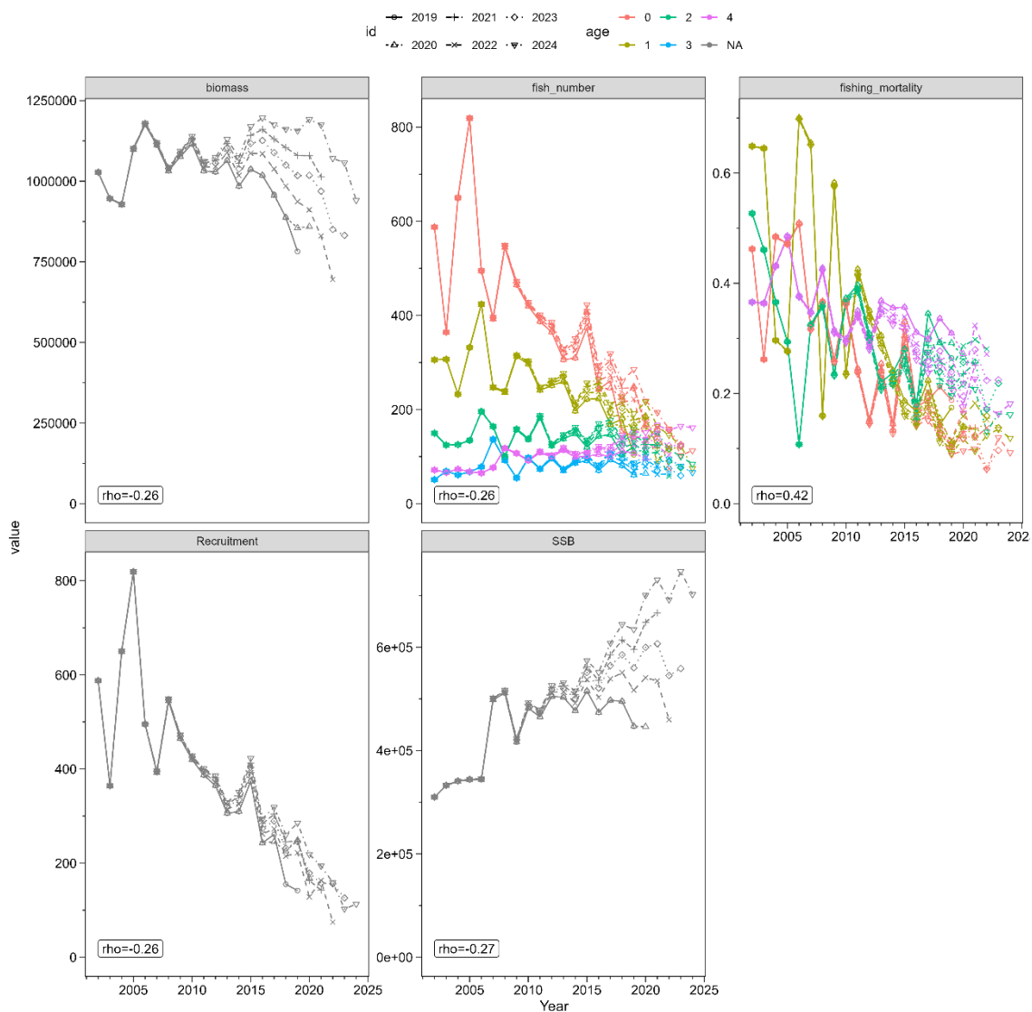
補足図 4-7. 3 海域独立した 1 歳魚資源量指標値を用いたチューニング VPA (独立指数 VPA) におけるレトロスペクティブ解析の結果
