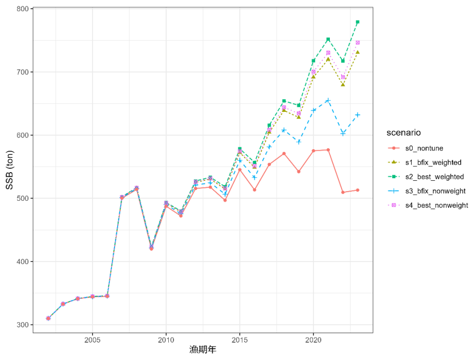
資料図 10-2. 試算結果の比較（親魚量）。S0：チューニングなし S1：検討 1、S2：検討 2、S3：検討 3、S4：検討 4。各検討の条件は補足表 10-1 を参照。
