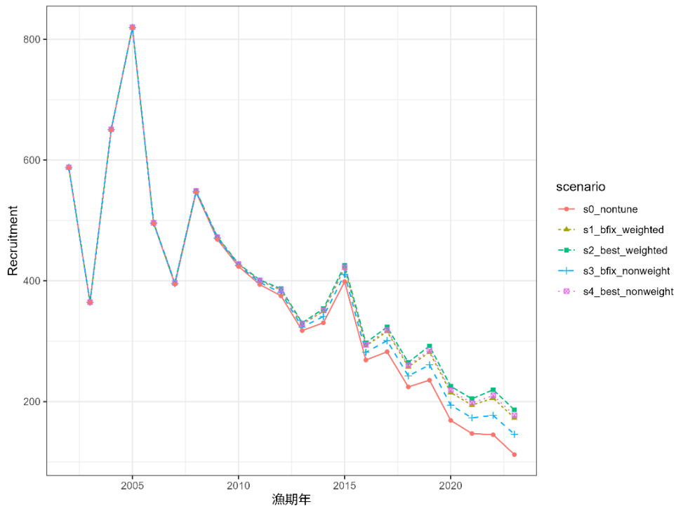
資料図 10-3. 試算結果の比較 (0歳資源尾数) S0 : チューニングなし。S1 : 検討1、S2 : 検討2、S3 : 検討3、S4 : 検討4。各検討の条件は補足表 10-1 を参照。
