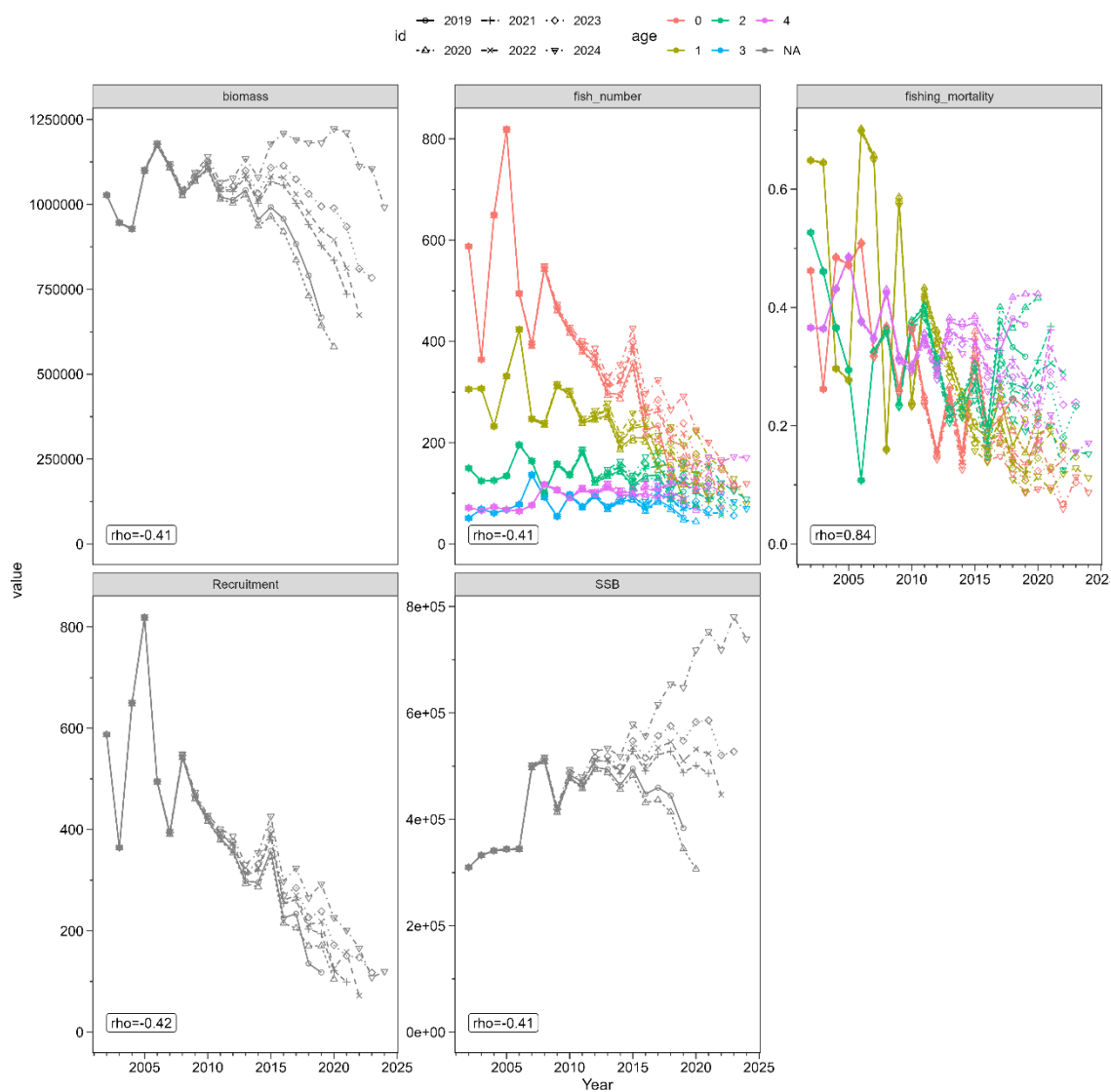
補足図 4-8. 3 海域統合 1 歳魚資源量指標値を用いたチューニング VPA (統合指数 VPA) におけるレトロスペクティブ解析の結果
