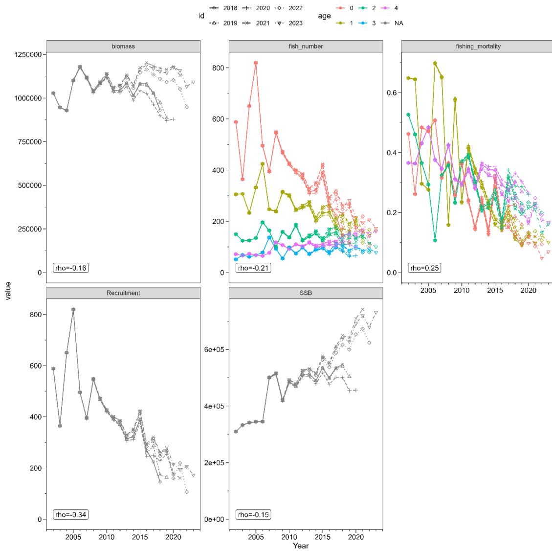
資料図 10-10. 検討 1 (最尤法、b 推定なし) におけるレトロスペクティブ解析の結果
