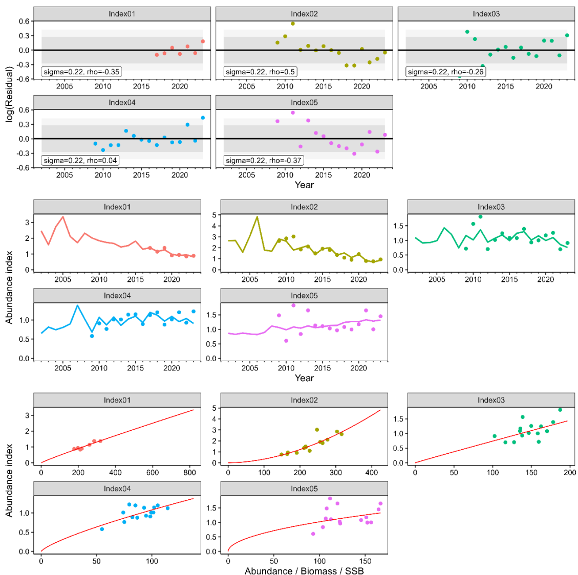
資料図 10-8. 検討 4 (最小二乗法、 b 推定あり) における残差プロット、指標値 (○) と予測値 (実線)、各年齢の指標値と年齢別資源尾数との相関。残差プロットのダークグレーは 80%信頼区間。対数残差には、尤度 ( \sigma : sigma)、Mohn's rho ( \rho ) を示した。 \rho のアスタリスクは自己相関係数が有意に大きい場合を示す。Index01: 0 歳 CPUE、Index02: 1 歳 CPUE、Index03: 2 歳 CPUE、Index04: 3 歳 CPUE、Index05: 4 歳以上 CPUE。
