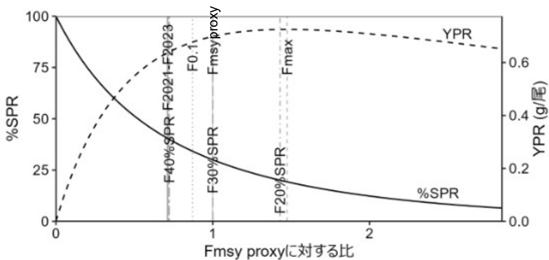
図 4-8. F と YPR、SPR の関係
