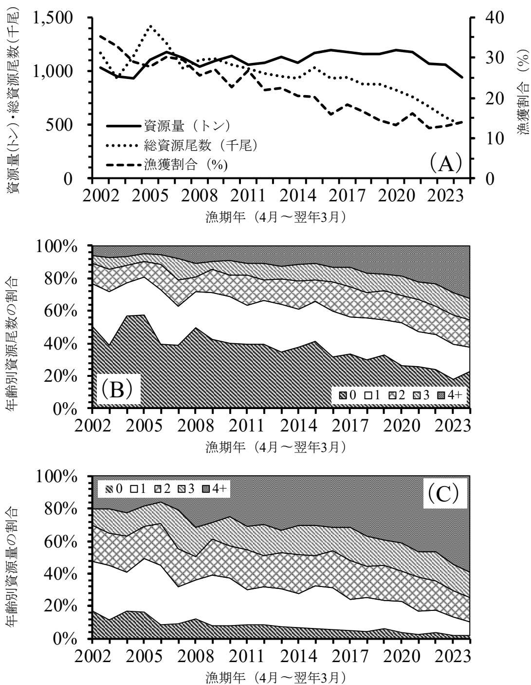
図 4-4. 資源量・総資源尾数・漁獲割合の推移 (A)、年齢別資源尾数の割合 (B)、年齢別資源量の割合 (C)
