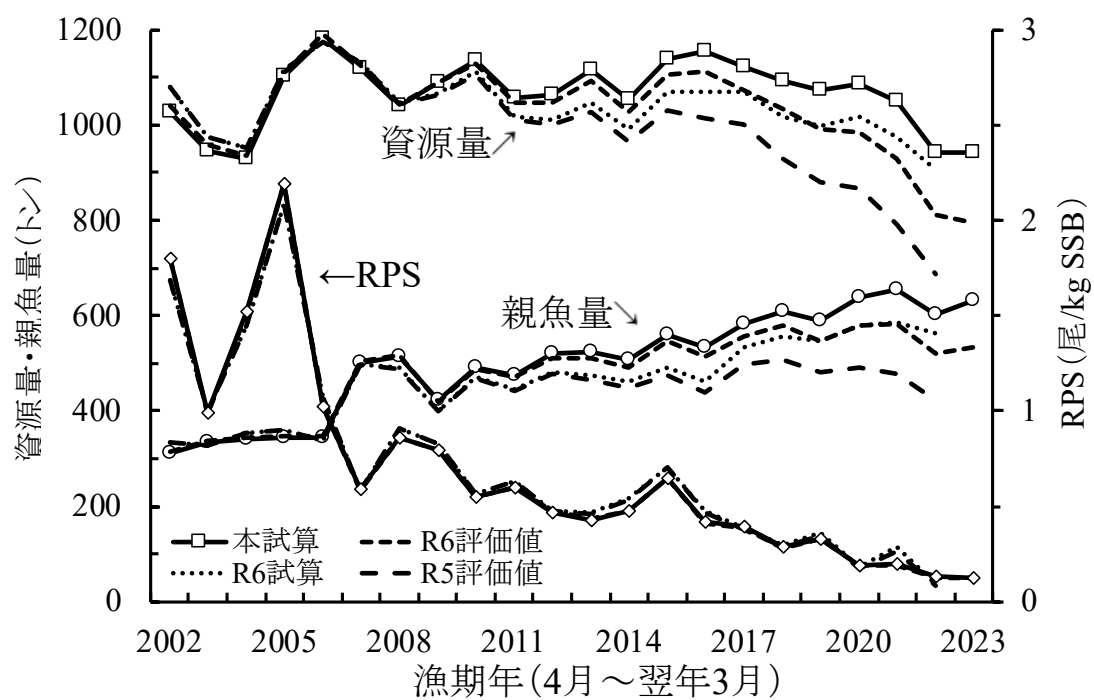
補足図 10-2. 海域別年齢別 CPUE を用いた全年齢チューニング VPA の試算結果。実線・ マーカー付：本試算、破線：R6 評価値、点線：R6 試算、大破線：R5 評価値。
