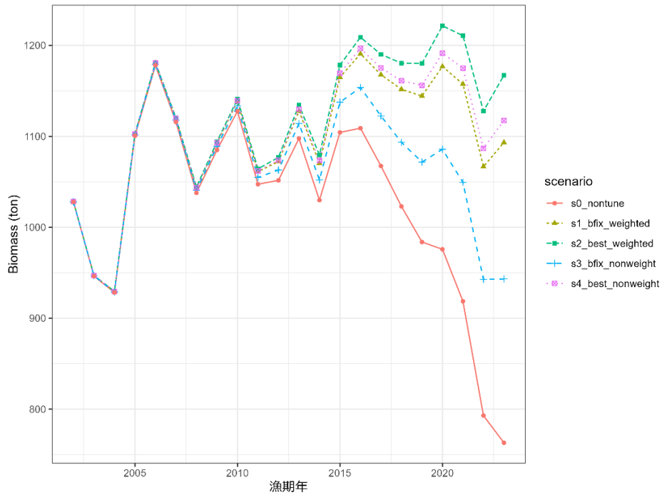
資料図 10-1. 試算結果の比較（資源量） S0：チューニングなし。S1：検討 1、S2：検討 2、S3：検討 3、S4：検討 4。各検討の条件は補足表 10-1 を参照。2、S3:検討 3、S4：検討 4。各検討の条件は補足表 10-1 を参照。
