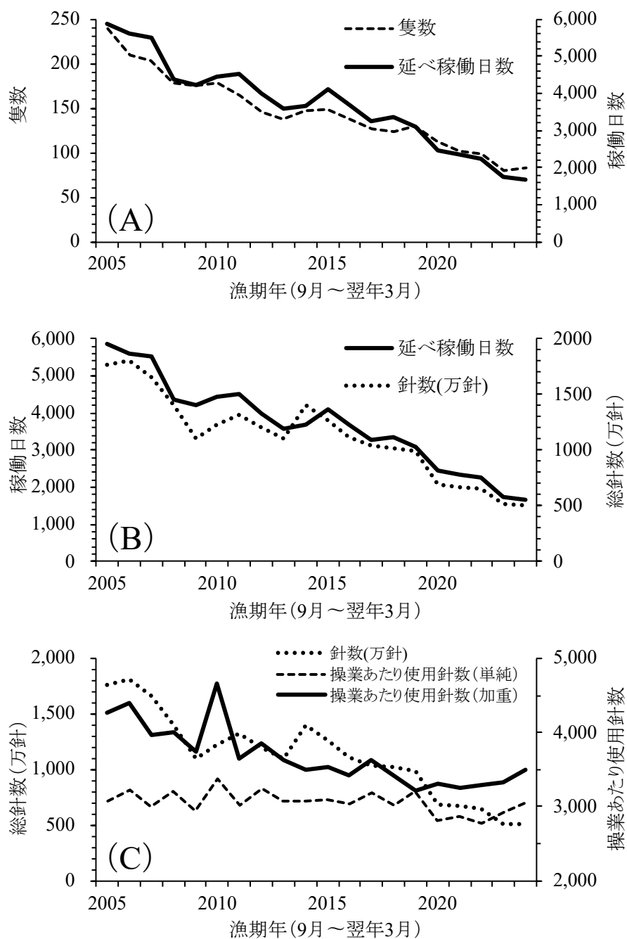
図 3-4. 九州・山口北西海域の 0 歳以上を対象としたはえ縄の努力量 (A) 各漁期年 (9 月～翌年 3 月) 中の稼働隻数と稼働日数、(B) 稼働日数と総使用針数 (単位: 万針)、(C) 総使用針数 (万針) に対する、操業あたり使用針数。破線: 単純平均、実線: 船別集計に基づく稼働日数に対する加重平均。
