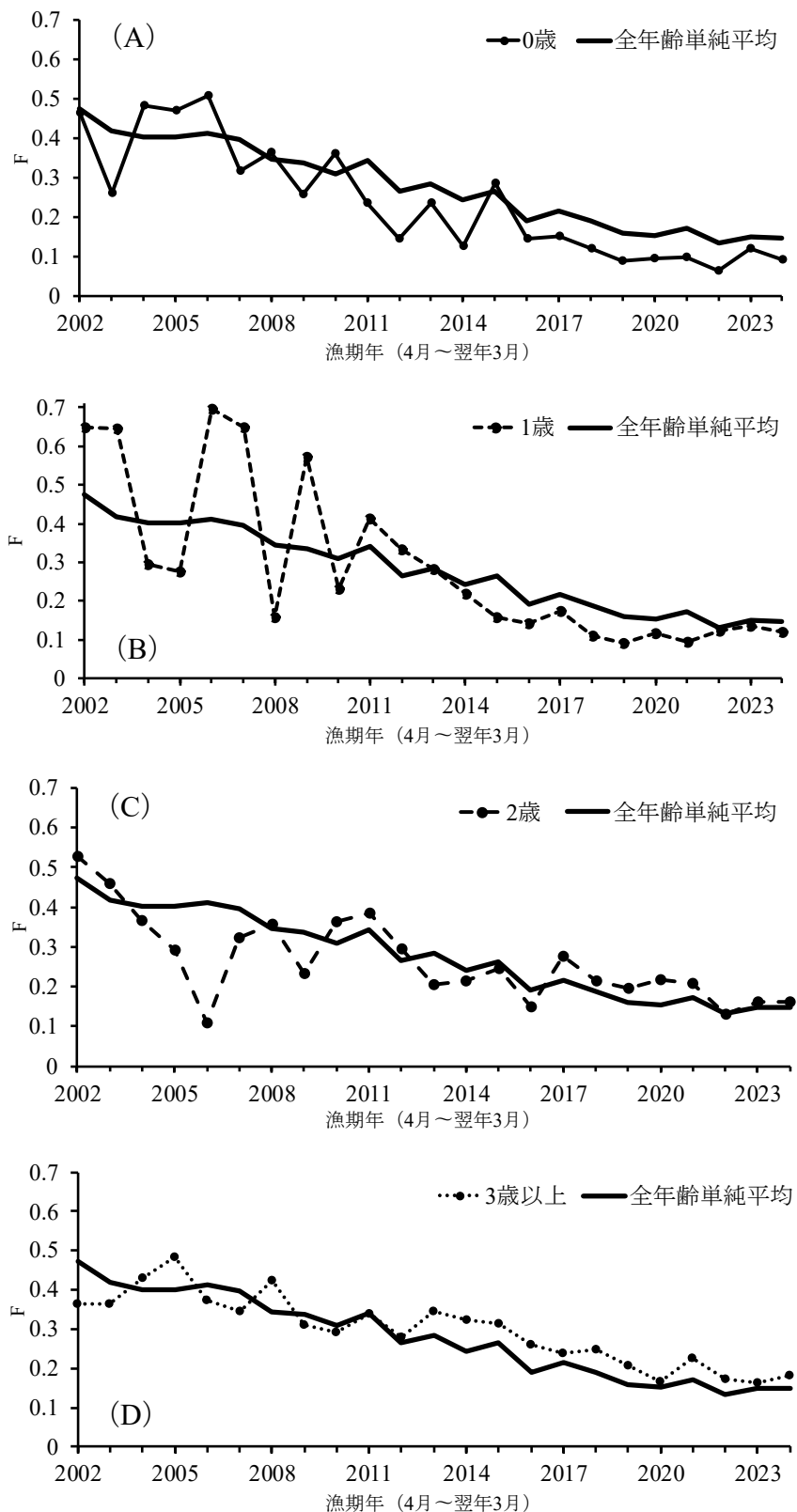
図 4-6. 各年齢の F と、F の全年齢平均の推移 (A) 0 歳、(B) 1 歳、(C) 2 歳、(D) 3 歳以上。4 歳以上は 3 歳 F と同じと仮定。
