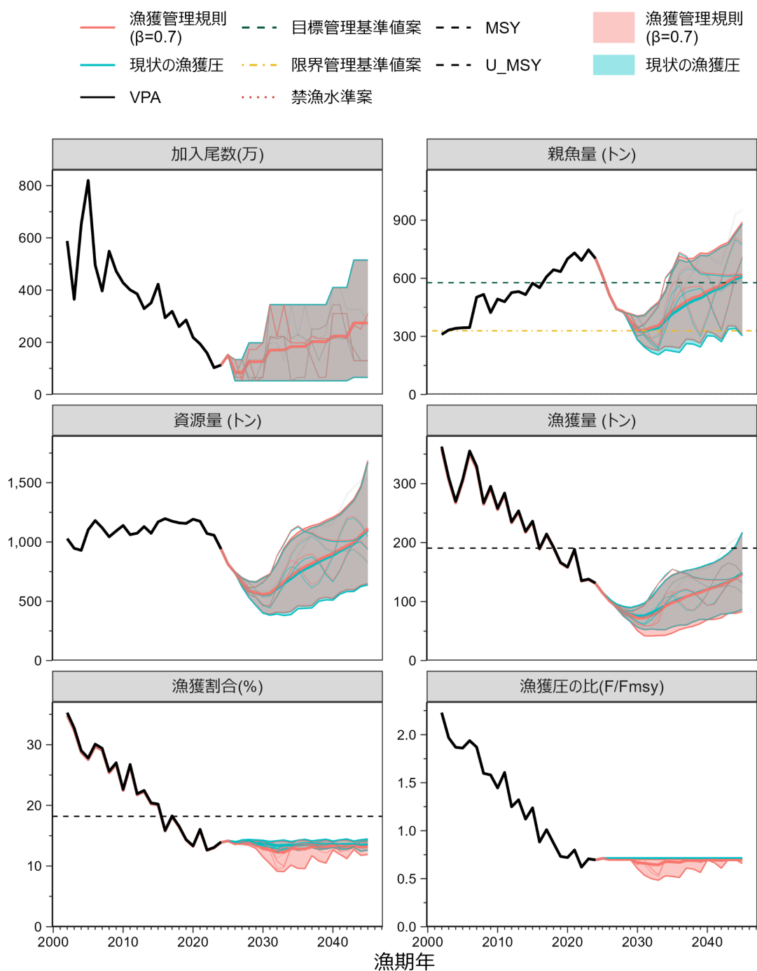
補足図 7-5. 漁獲管理規則案を用いた場合（赤線）と現状の漁獲圧での将来予測（青色） （2026年漁期以降を天然のみの加入の場合、2025年漁期は、2019～2023年漁期の平均放流加入尾数を仮定（仮定3））太実線は平均値、網掛けはシミュレーション結果の90%が含まれる予測区間、細線は5通りの将来予測の例示である。親魚量の図の緑破線は目標管理基準値案、黄一点鎖線は限界管理基準値案、赤点線は禁漁水準案を示す。漁獲割合の図の破線は U_{msy} を示す。漁獲管理規則での調整係数 \beta には 0.7 を用いた。
