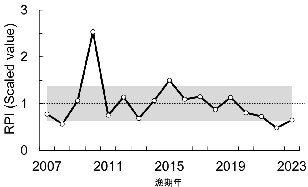
補足図 10-4. 産卵親魚来遊指標値を用いた天然資源尾数の加入指標の算出
