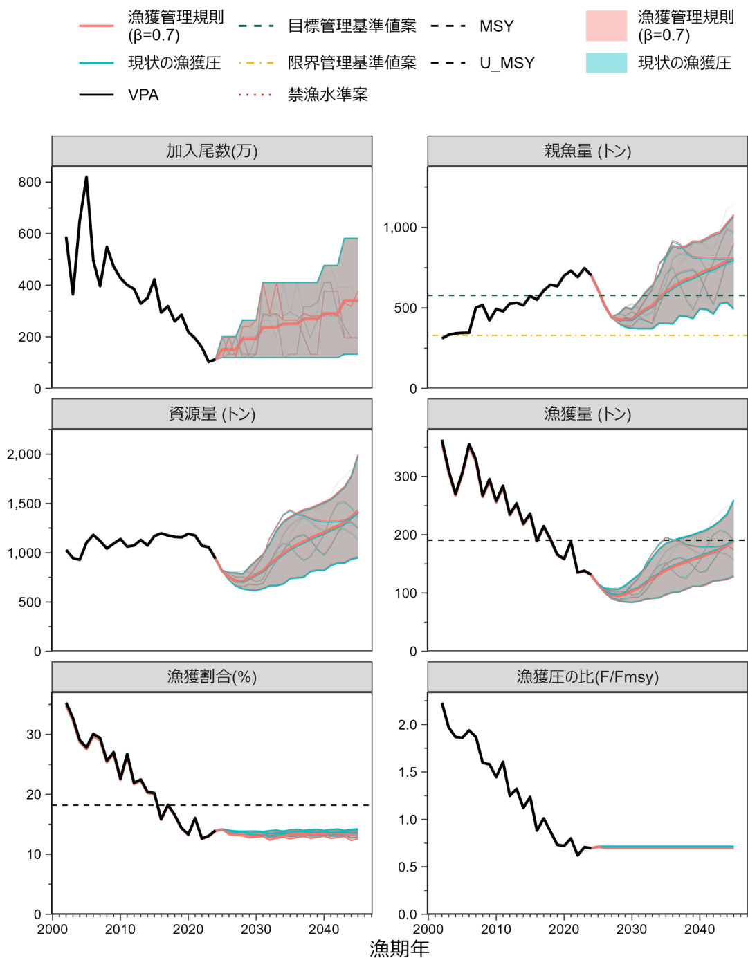
補足図 7-7. 漁獲管理規則案を用いた場合（赤線）と現状の漁獲圧での将来予測（青色） （2025 年漁期以降は、2019～2023 年漁期の平均放流加入尾数を仮定（仮定 5）） 太 実線は平均値、網掛けはシミュレーション結果の 90%が含まれる予測区間、細線は 5 通りの将来予測の例示である。親魚量の図の緑破線は目標管理基準値案、黄一点鎖線 は限界管理基準値案、赤点線は禁漁水準案を示す。漁獲割合の図の破線は U_{msy} を示 す。漁獲管理規則での調整係数 \beta には 0.7 を用いた。
