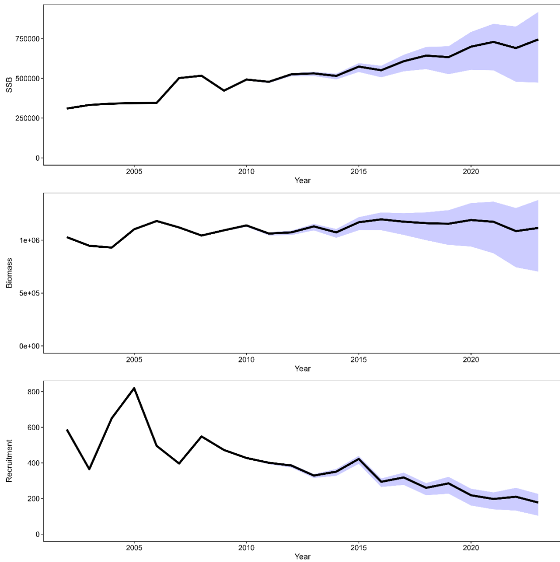
資料図 10-17. 検討 4 (最小二乗法、b 推定あり) におけるブートストラップ信頼区間推定結果 紫色の影の範囲は 95%信頼区間を示す。上から順に、親魚量 (単位: トン)、資源量 (単位: トン)、0 歳資源尾数 (単位: 千尾)。
