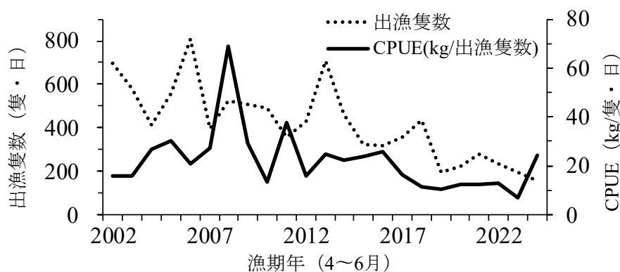
図 3-7. 備讃瀬戸における標本漁協の 1 歳以上 (1 kg 以上) を対象とした袋待網の努力量と単純 CPUE の推移 2019 年以降は一標本漁協について出漁隻数、単純 CPUE を算出。
