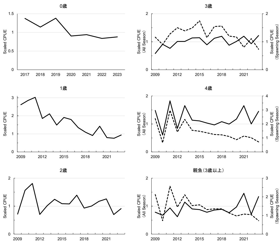
補足図 10-1. 海域別年齢別 CPUE。横軸は漁期年（4 月～翌年 3 月）。チューニングに適用した期間（2009～2023 年漁期、0 歳は 2017～2023 年漁期）を示す。実線は通年、破線は産卵期（4～7 月）の結果。
