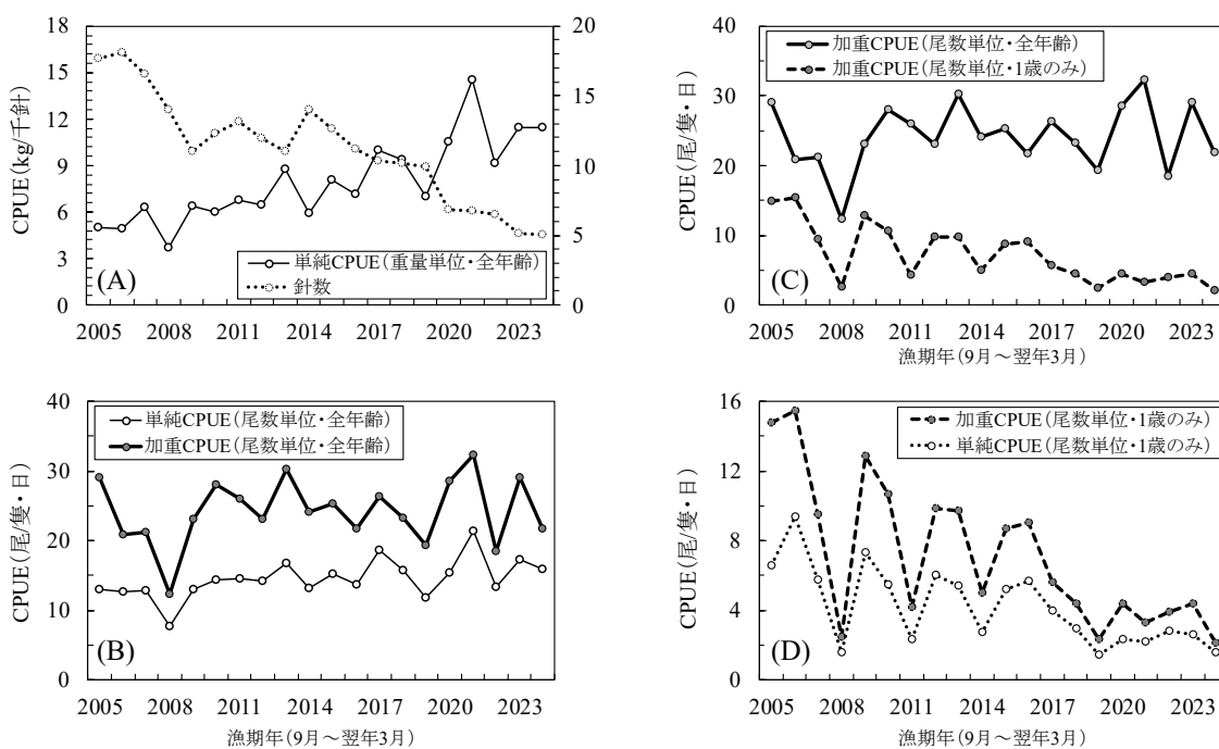
補足図 4-1. 九州・山口北西海域とらふぐはえ縄漁獲成績報告書から抽出した、日本海中西部・東シナ海におけるはえ縄の資源量指標値 (A) : 過去の資源評価票において提示してきた漁獲努力量 (針数) と単純 CPUE、(B) : 尾数単位での単純 CPUE と加重 CPUE、(C) : 全年齢と 1 歳魚の加重 CPUE の比較、(D) : 1 歳魚の加重 CPUE と単純 CPUE の比較。
