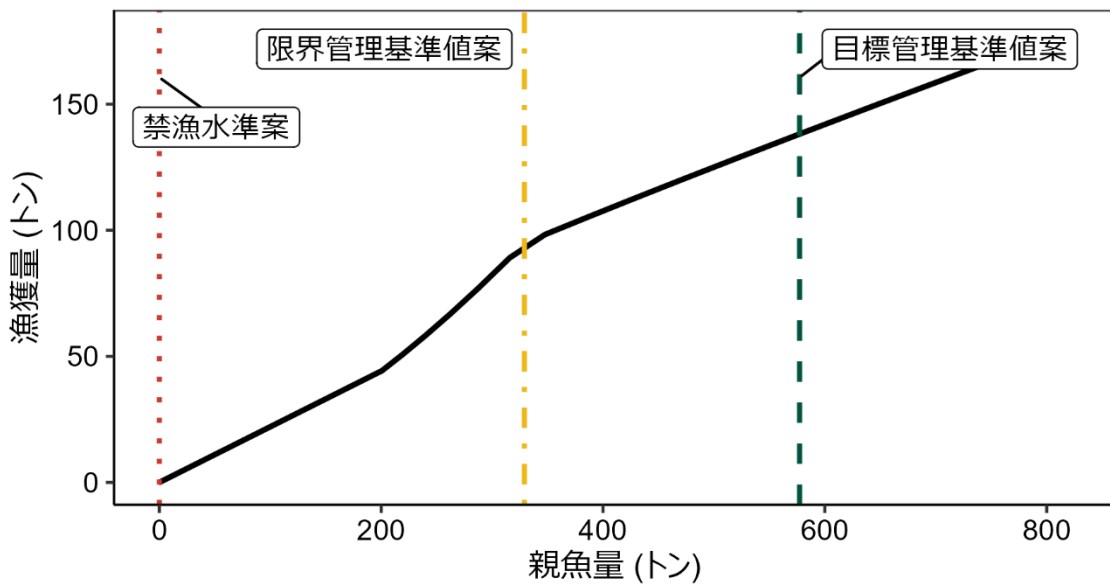
補足図 7-3. 漁獲管理規則案
