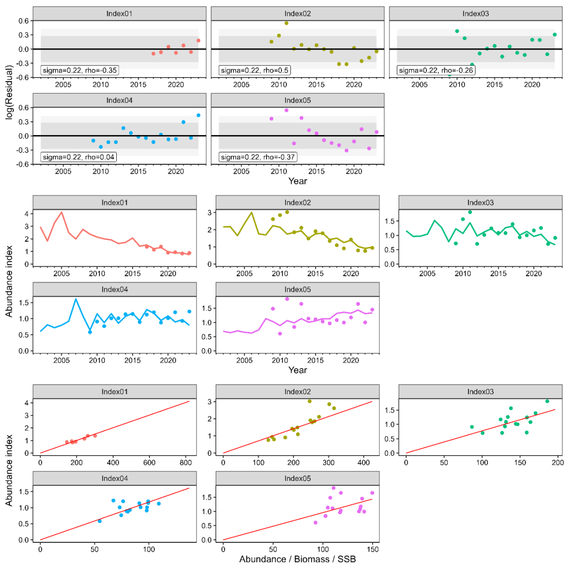
資料図 10-7. 検討 3 (最小二乗法、 b 推定なし) における残差プロット、指標値 (○) と予測値 (実線)、各年齢の指標値と年齢別資源尾数との相関 残差プロットのダークグレーは 80%信頼区間。対数残差には、尤度 ( \sigma : \sigma )、Mohn's rho ( \rho ) を示した。 \rho のアスタリスクは自己相関係数が有意に大きい場合を示す。Index01: 0 歳 CPUE、Index02: 1 歳 CPUE、Index03: 2 歳 CPUE、Index04: 3 歳 CPUE、Index05: 4 歳以上 CPUE。
