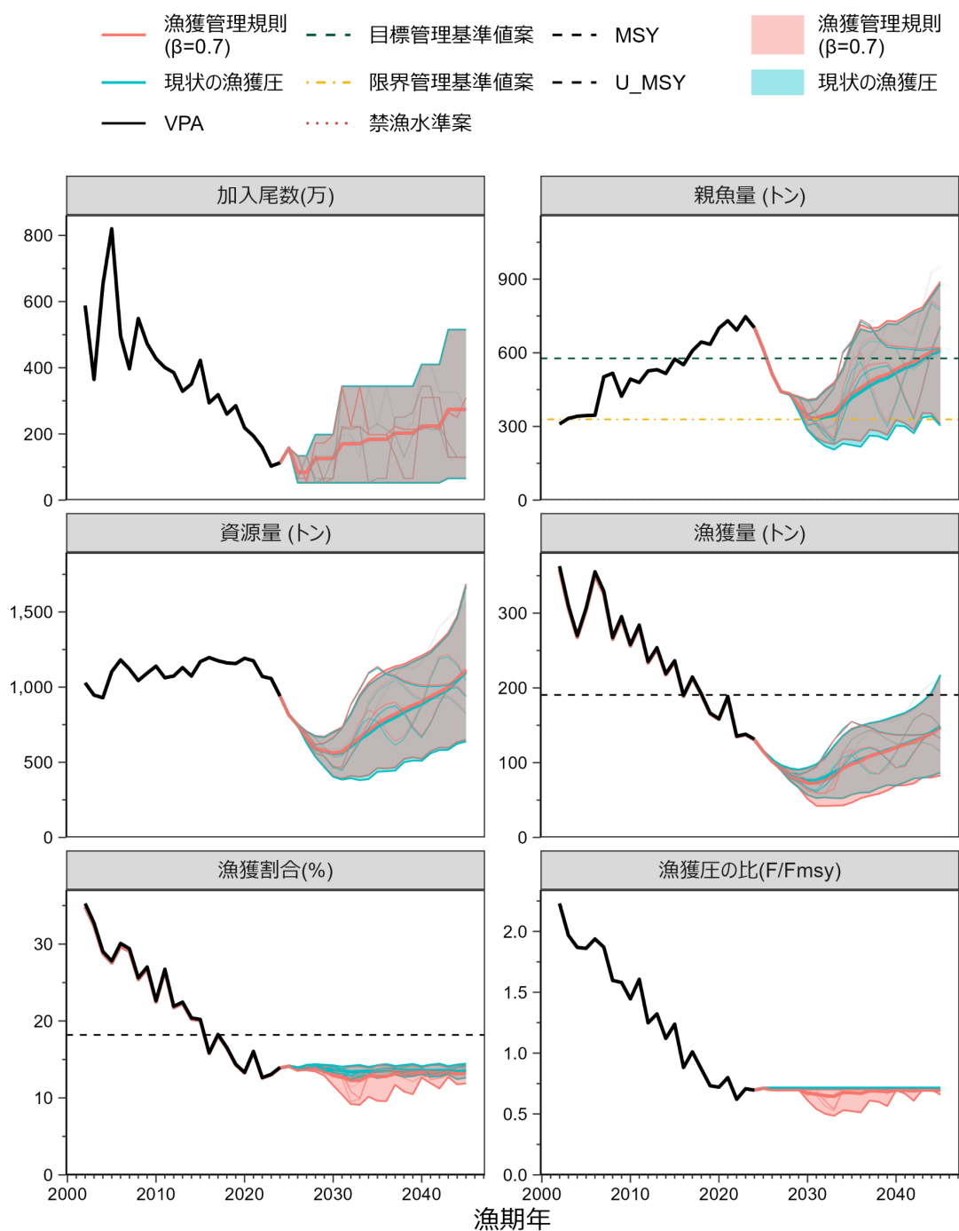
補足図 7-4. 漁獲管理規則案を用いた場合（赤線）と現状の漁獲圧での将来予測（青色） （2026 年漁期以降を天然のみの加入の場合、2025 年漁期は、2016～2020 年漁期の平均放流加入尾数を仮定（仮定 2））太実線は平均値、網掛けはシミュレーション結果の 90%が含まれる予測区間、細線は 5 通りの将来予測の例示である。親魚量の図の緑破線は目標管理基準値案、黄一点鎖線は限界管理基準値案、赤点線は禁漁水準案を示す。漁獲割合の図の破線は U_{msy} を示す。漁獲管理規則での調整係数 \beta には 0.7 を用いた。
