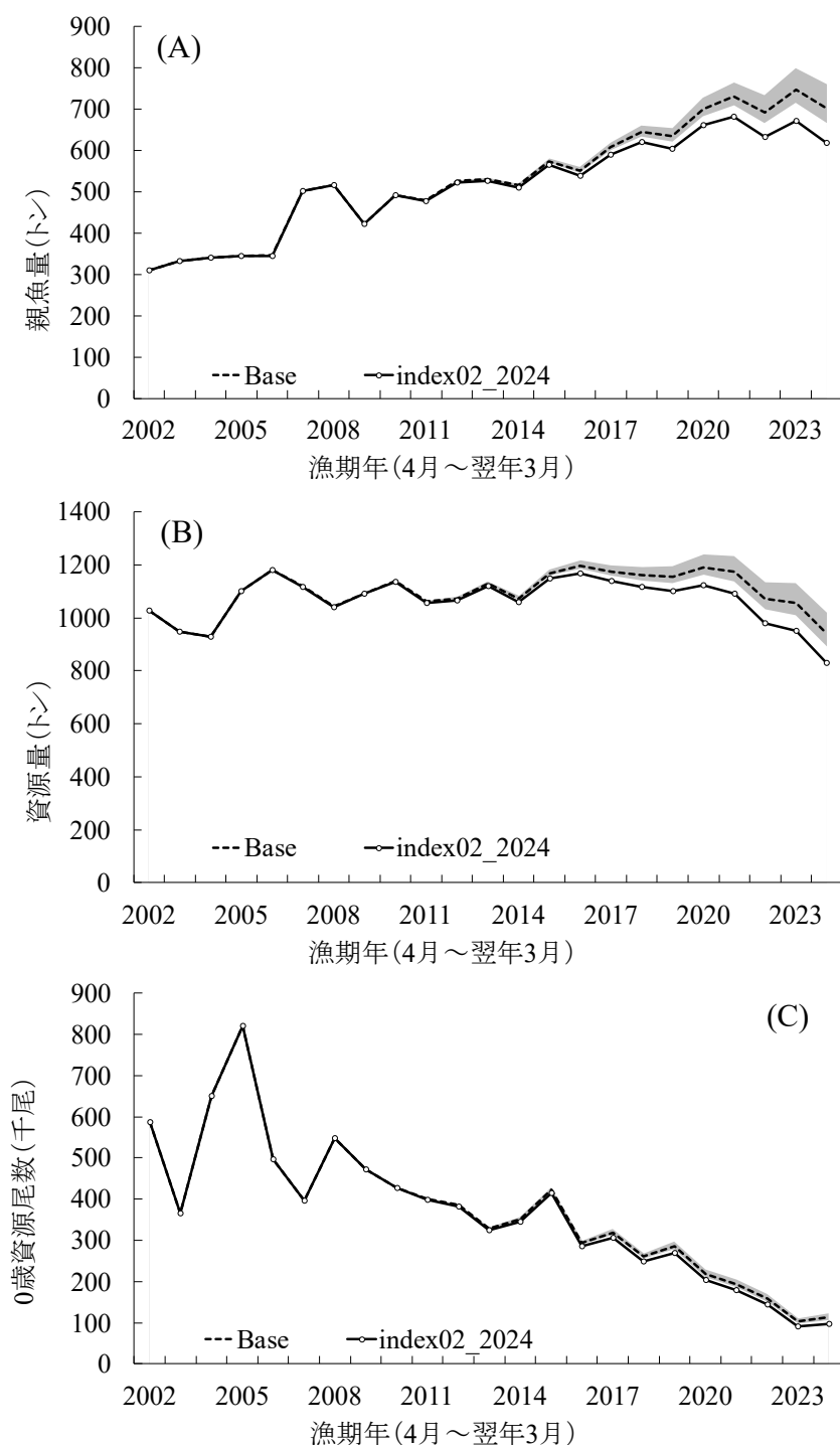
補足図 4-9. 3 海域独立した 1 歳魚資源量指標値を用いたチューニング VPA (独立指数 VPA) に対する、ジャックナイフ法によるチューニング指標値の影響解析結果。Base (破線) は各年の指標値を全て使用した場合。実線：2024 年漁期の index02 のみ除外。グレー帯は、index02 の 2024 年漁期値以外の指標値を除外した場合の各漁期年の最大値～最小値の幅を示す。(A) 親魚量 (単位：トン)、(B) 資源量 (単位：トン)、(C) 0 歳資源尾数 (単位：千尾)。
