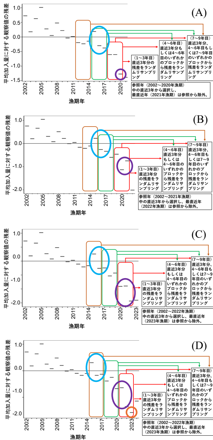
補足図 7-1. 将来予測における加入尾数の仮定に用いるブロックバックワードリサンプリングの模式図 (A) 研究機関会議で用いられた加入尾数の残差 (参照年: 2002~2020年漁期)、(B) R5 年度評価での加入尾数に基づく残差 (参照年: 2002~2021年漁期)。(C) R6 年度評価での加入尾数に基づく残差 (参照年: 2002~2022年漁期)。(D) 本年度評価 (参照年: 2002~2023年漁期)。過去の加入状況は古いブロックに移るため、参照されにくく (例: 水色枠内)、近年の加入状況 (紫枠、橙枠内) が参照され、近年の加入状況を反映した予測が可能となる。
