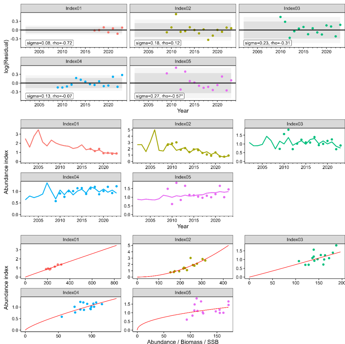
資料図 10-6. 検討 2 (最尤法、b 推定あり) における残差プロット、指標値 (○) と予測値 (実線)、各年齢の指標値と年齢別資源尾数との相関。残差プロットのダークグレーは 80%信頼区間、ライトグレーは 95%信頼区間を示す。対数残差には、尤度 ( \sigma : sigma)、Mohn's rho ( \rho ) を示した。rho のアスタリスクは自己相関係数が有意に大きい場合を示す。Index01 : 0 歳 CPUE、Index02 : 1 歳 CPUE、Index03 : 2 歳 CPUE、Index04 : 3 歳 CPUE、Index05 : 4 歳以上 CPUE。
