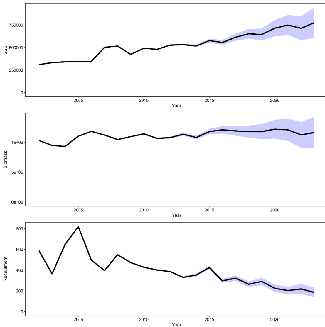
資料図 10-15. 検討 2 (最尤法、 b 推定あり) におけるブートストラップ信頼区間推定結果 紫色の影の範囲は 95%信頼区間を示す。上から順に、親魚量 (単位: トン)、資源量 (単位: トン)、0 歳資源尾数 (単位: 千尾)。
