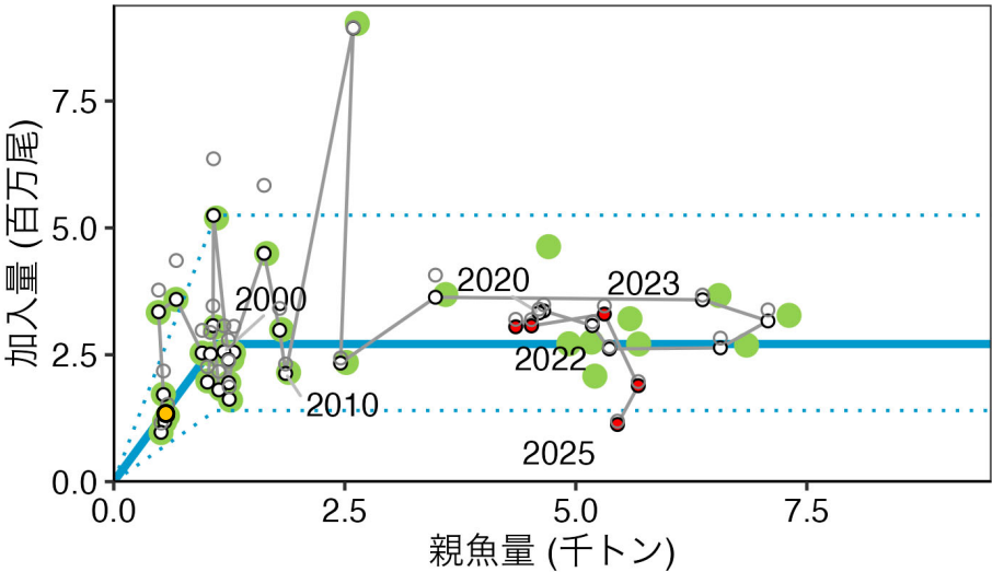
図6 再生産関係
