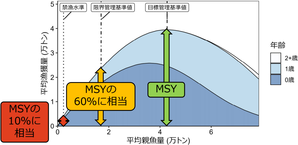
図7 管理基準値
