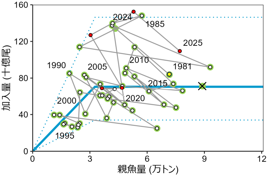
図6 再生産関係
