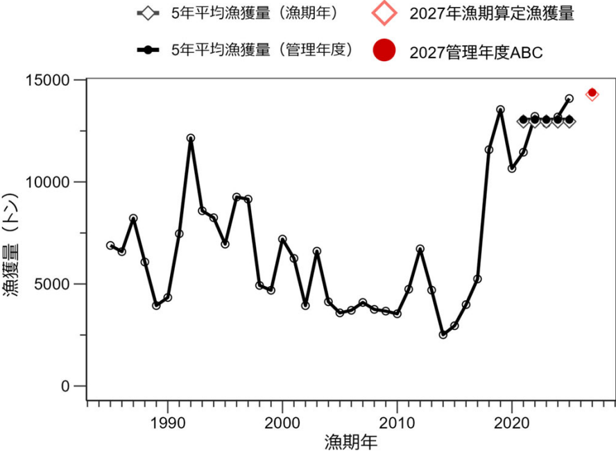
図6 漁獲量の推移と2027管理年度のABC
