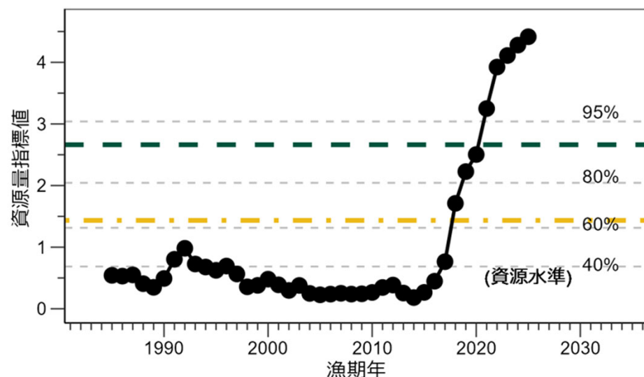
図4 資源水準および管理基準値
