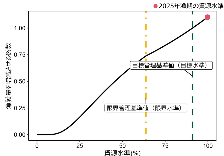
図5 漁獲シナリオ
