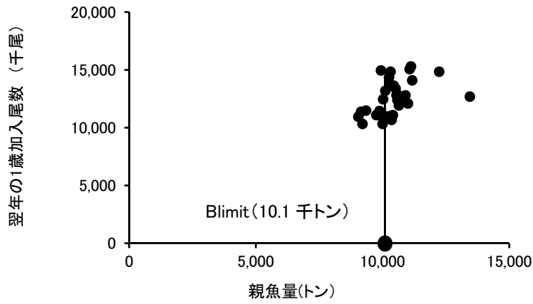
図 12. 再生産関係
